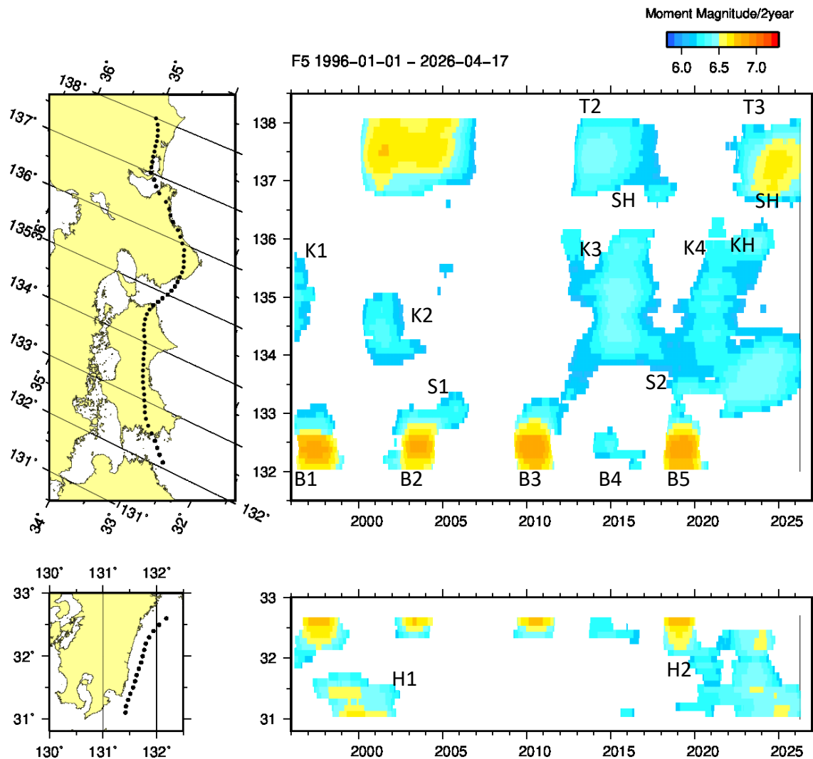
第2図 長期的スロースリップの規模分布 (1996年～2026年4月) 2年間あたりの変化量から推定したモーメントマグニチュード。
