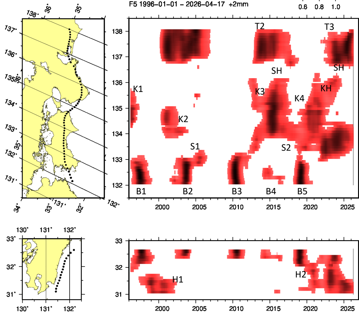
第1図 長期的スロースリップ客観検知図（1996年～2026年4月）
