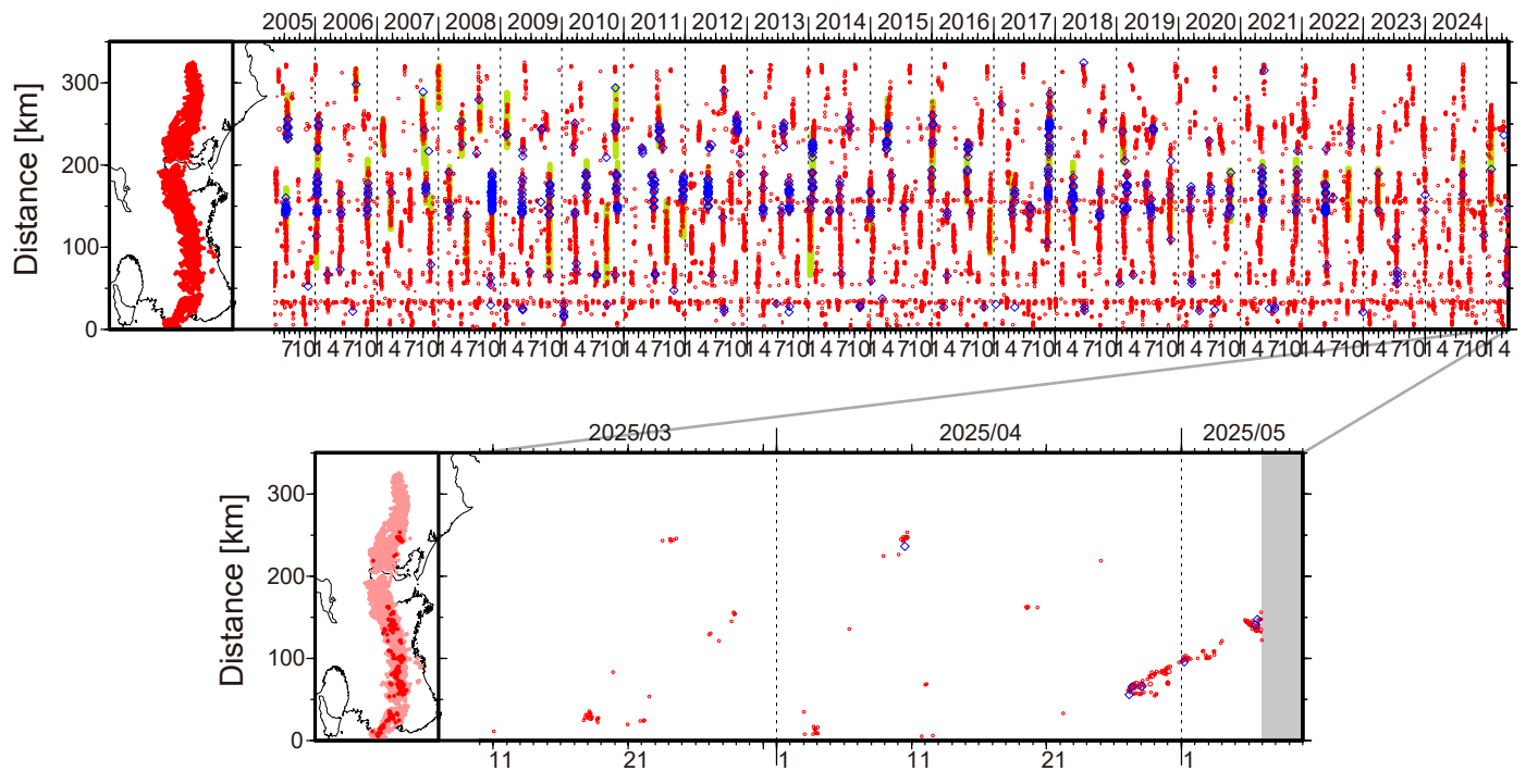
図 1. 紀伊半島・東海地域における 2005 年 5 月～2025 年 5 月 6 日までの深部低周波微動の時空間分布(上図)．赤丸はエンベロープ相関・振幅ハイブリッド法 (Maeda and Obara, 2009) およびクラスタ処理 (Obara et al., 2010) によって 1 時間毎に自動処理された微動分布の重心である．青菱形は周期 20 秒に卓越する超低周波地震 (Ito et al., 2007) である．黄緑色の太線はこれまでに検出された短期的スロースリップイベント (SSE) を示す．下図は 2025 年 4 月を中心とした期間の拡大図である．4 月 27 日頃からは奈良県南部で微動活動が開始し、北東方向への活動域の移動が 5 月 4 日頃までみられた．5 月 5 日 17:05 頃に三重県北部深さ約 18km で発生した M2.8 の地震 (Hi-net 暫定値) 後の 17:10 過ぎからは三重県中部で活動が活発化している．4 月 3～4 日頃には和歌山県中部において小規模な活動がみられた．4 月 10 日頃には愛知県中部において、4 月 19～20 日頃には三重県北部において、それぞれごく小規模な活動がみられた．
