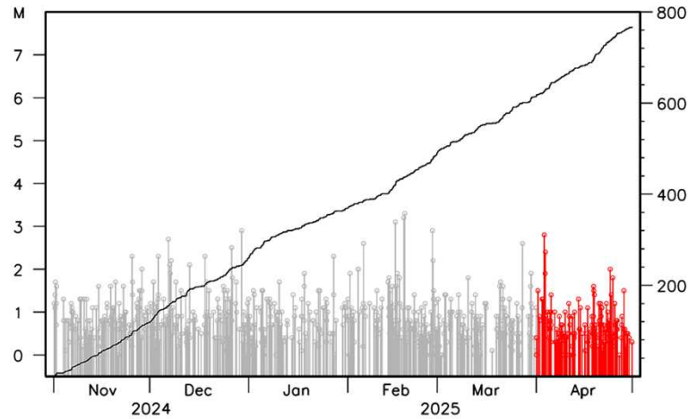
領域c内(四国)
