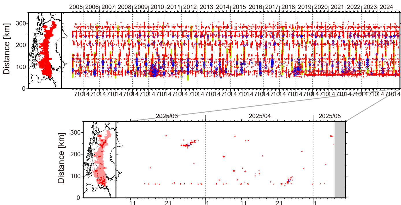
図 1. 四国における 2005 年 5 月～ 2025 年 5 月 6 日までの深部低周波微動の時空間分布 (上図). 赤丸はエンベロープ相関・振幅ハイブリッド法 (Maeda and Obara, 2009) およびクラスター処理 (Obara et al., 2010) によって 1 時間毎に自動処理された微動分布の重心である. 青菱形は周期 20 秒に卓越する超低周波地震 (Ito et al., 2007) である. 黄緑色太線は、これまでに検出された短期的スロースリップイベント (SSE) を示す. 下図は 2025 年 4 月を中心とした期間の拡大図である. 4 月 22 ～ 25 日頃には豊後水道においてやや活発な活動がみられ、東方向への活動域の拡大がみられた. 4 月 8 ～ 9 日および 4 月 11 ～ 12 日頃には伊予灘付近で、4 月 12 日頃には香川・徳島県境付近で、それぞれごく小規模な微動活動がみられた. 5 月 5 日頃からは、香川県付近で微動活動が開始している.
