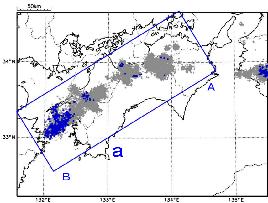
震央分布図（2019年4月1日～2025年5月1日、 深さ0～60km、Mすべて） 灰：2019年4月1日～2025年4月21日、 青：2025年4月22日以降
