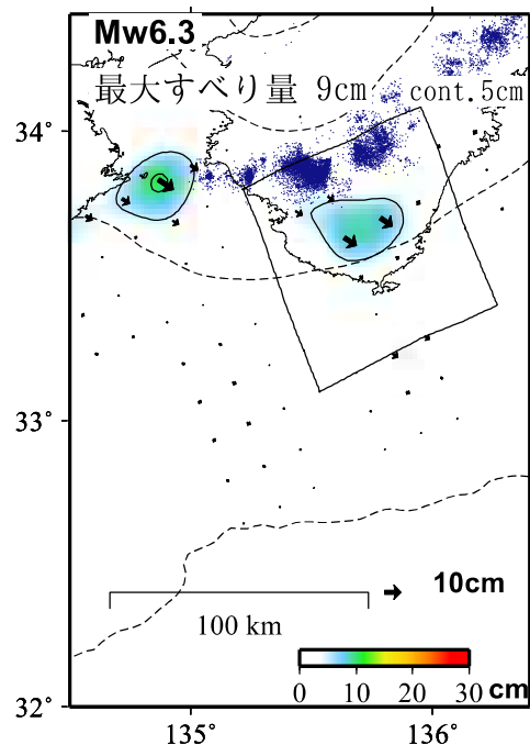
推定すべり分布 (2020-01-01/2025-03-09)
