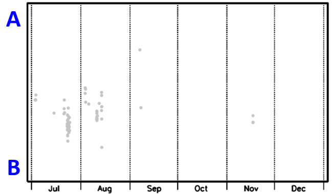
領域a内の時空間分布図(A-B投影) (2024年7月1日～2024年12月31日)
