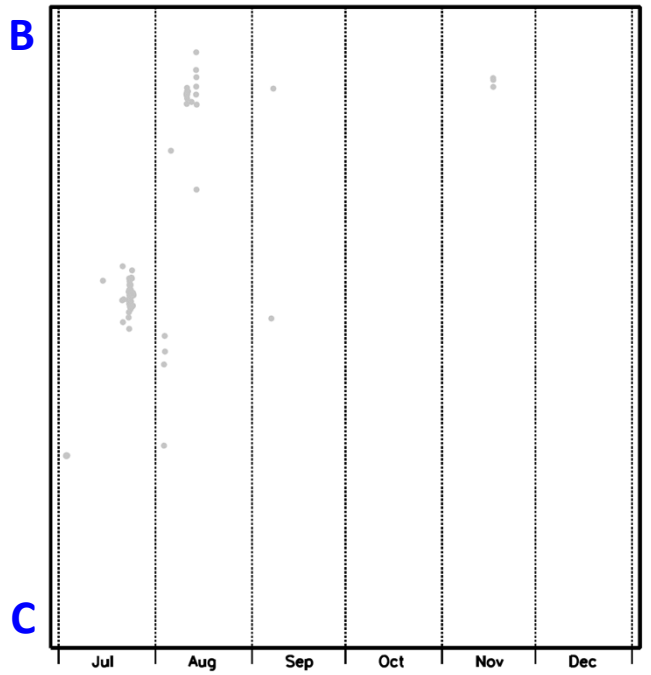
領域a内の時空間分布図(B-C投影) (2024年7月1日～2024年12月31日)
