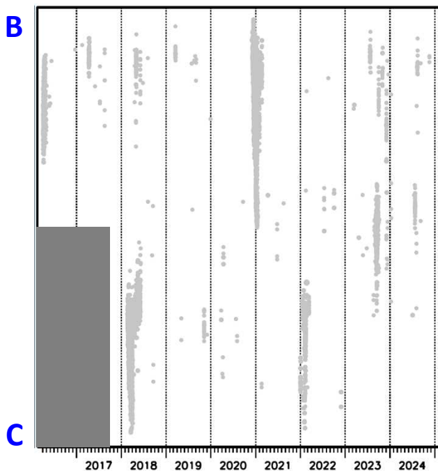
領域a内の時空間分布図(B-C投影) (2016年4月1日～2024年12月31日)
