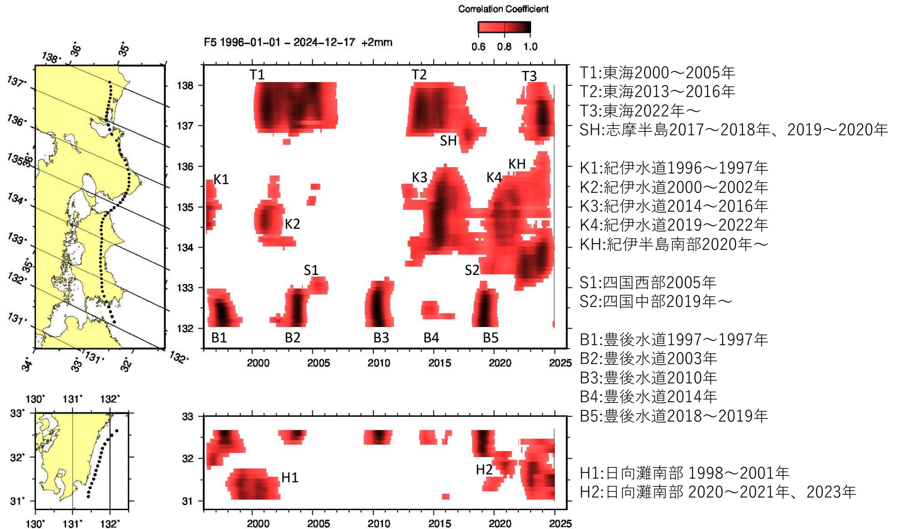
第1図 長期的スロースリップ客観検知図（1996年～2024年12月）
