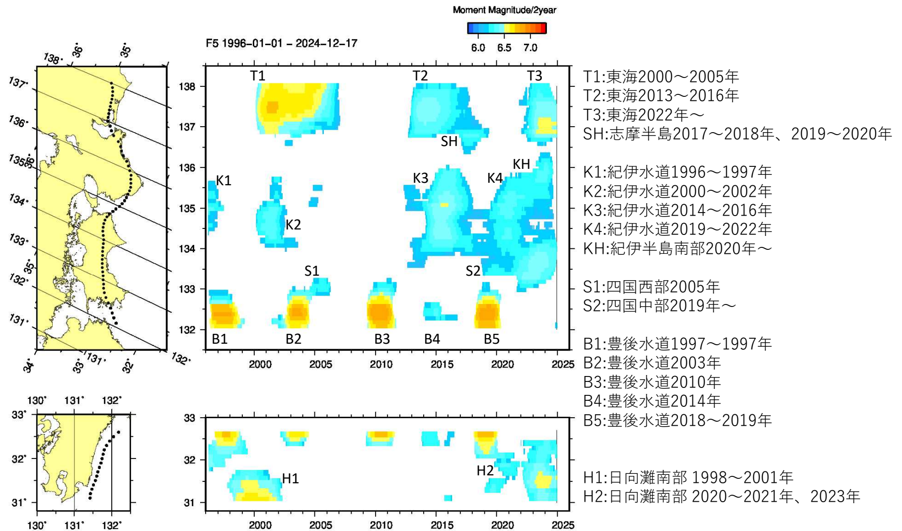
第2図 長期的スロースリップの規模分布（1996年～2024年12月） 2年間あたりの変化量から推定したモーメントマグニチュード。
