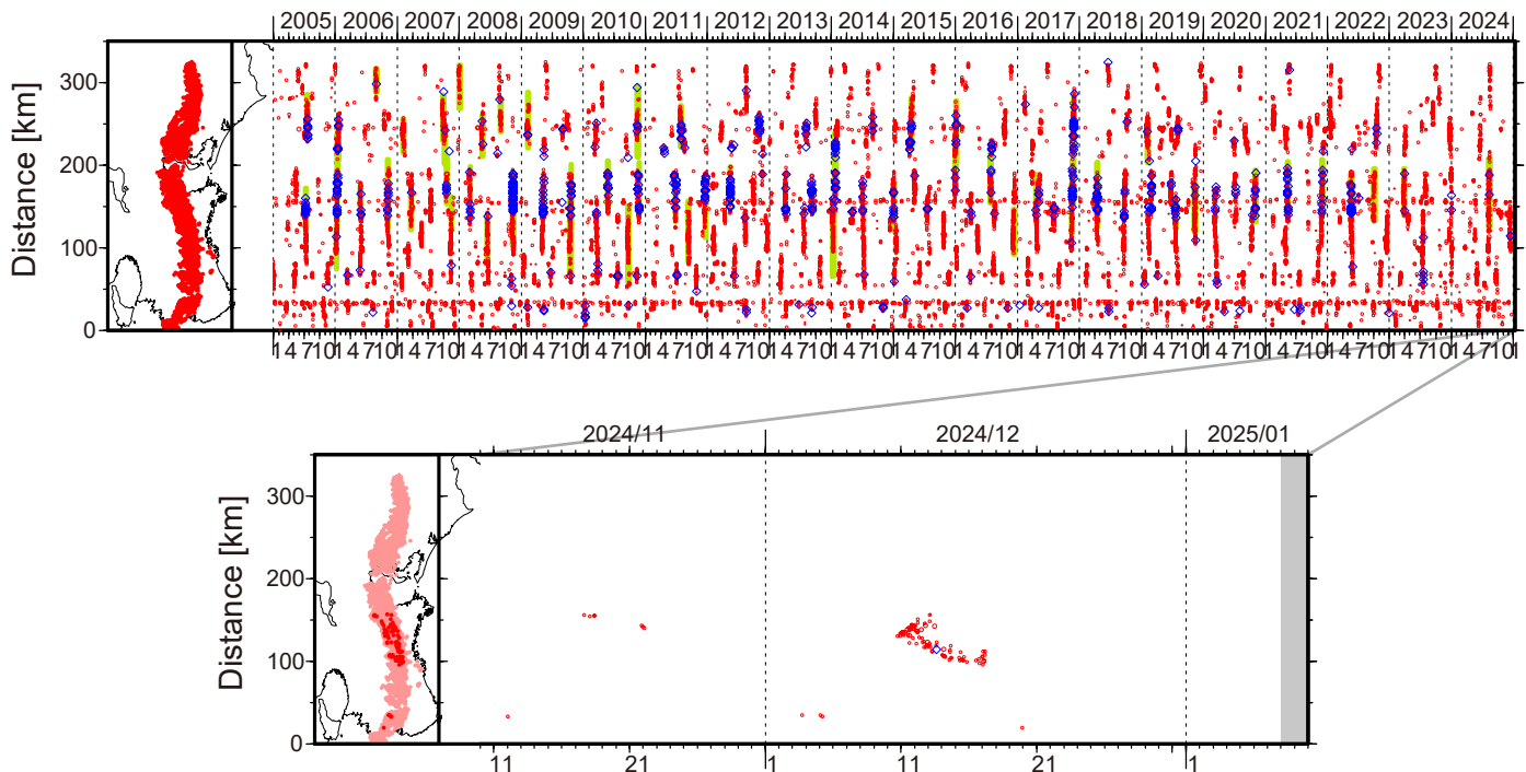
図1. 紀伊半島・東海地域における2005年1月～2025年1月7日までの深部低周波微動の時空間分布(上図)。赤丸はエンベロープ相関・振幅ハイブリッド法(Maeda and Obara, 2009)およびクラスタ処理(Obara et al., 2010)によって1時間毎に自動処理された微動分布の重心である。青菱形は周期20秒に卓越する超低周波地震(Ito et al., 2007)である。黄緑色の太線はこれまでに検出された短期的スロースリップイベント(SSE)を示す。下図は2024年12月を中心とした期間の拡大図である。12月10～17日頃には三重県中部から三重・奈良県境付近において、活発な微動活動がみられた。この活動は三重・奈良県境付近から開始し、13日頃まで北東・南西両方向への活動域の拡大がみられた。その後、南西方向への活動域の移動が17日頃までみられた。
