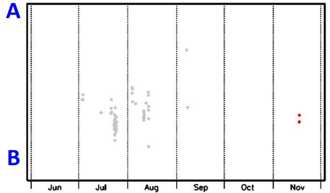
領域a内の時空間分布図(A-B投影) (2024年6月1日～2024年11月30日)
