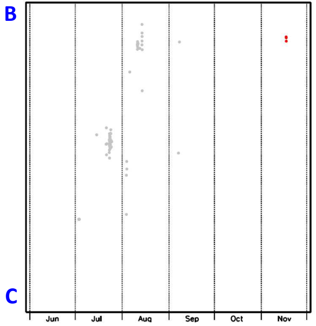
領域a内の時空間分布図(B-C投影) (2024年6月1日～2024年11月30日)
