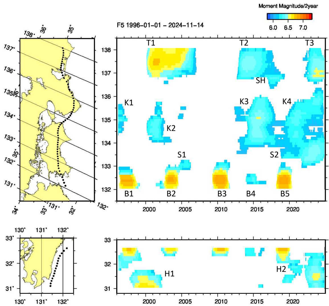
第2図 長期的スロースリップの規模分布 (1996年～2024年11月) 2年間あたりの変化量から推定したモーメントマグニチュード。
