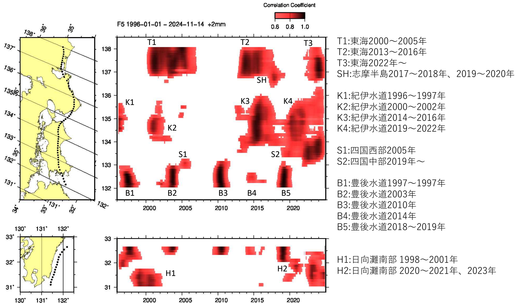
第1図 長期的スロースリップ客観検知図（1996年～2024年11月）
