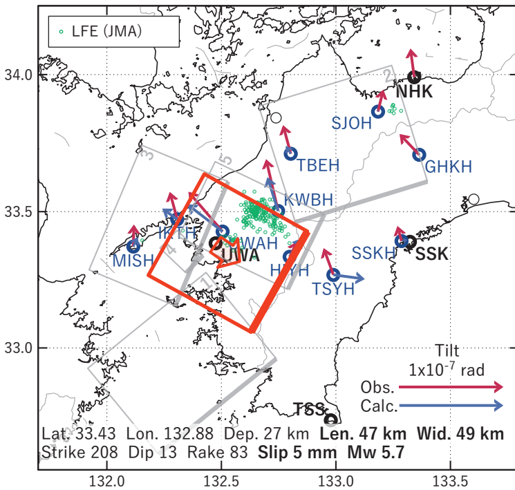
図6 2024/11/15PM-17の歪・傾斜変化(図5[A])を説明する断層モデル。
