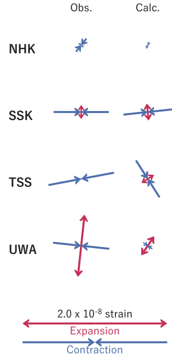
図6 2024/11/15PM-17の歪・傾斜変化(図5[A])を説明する断層モデル。
