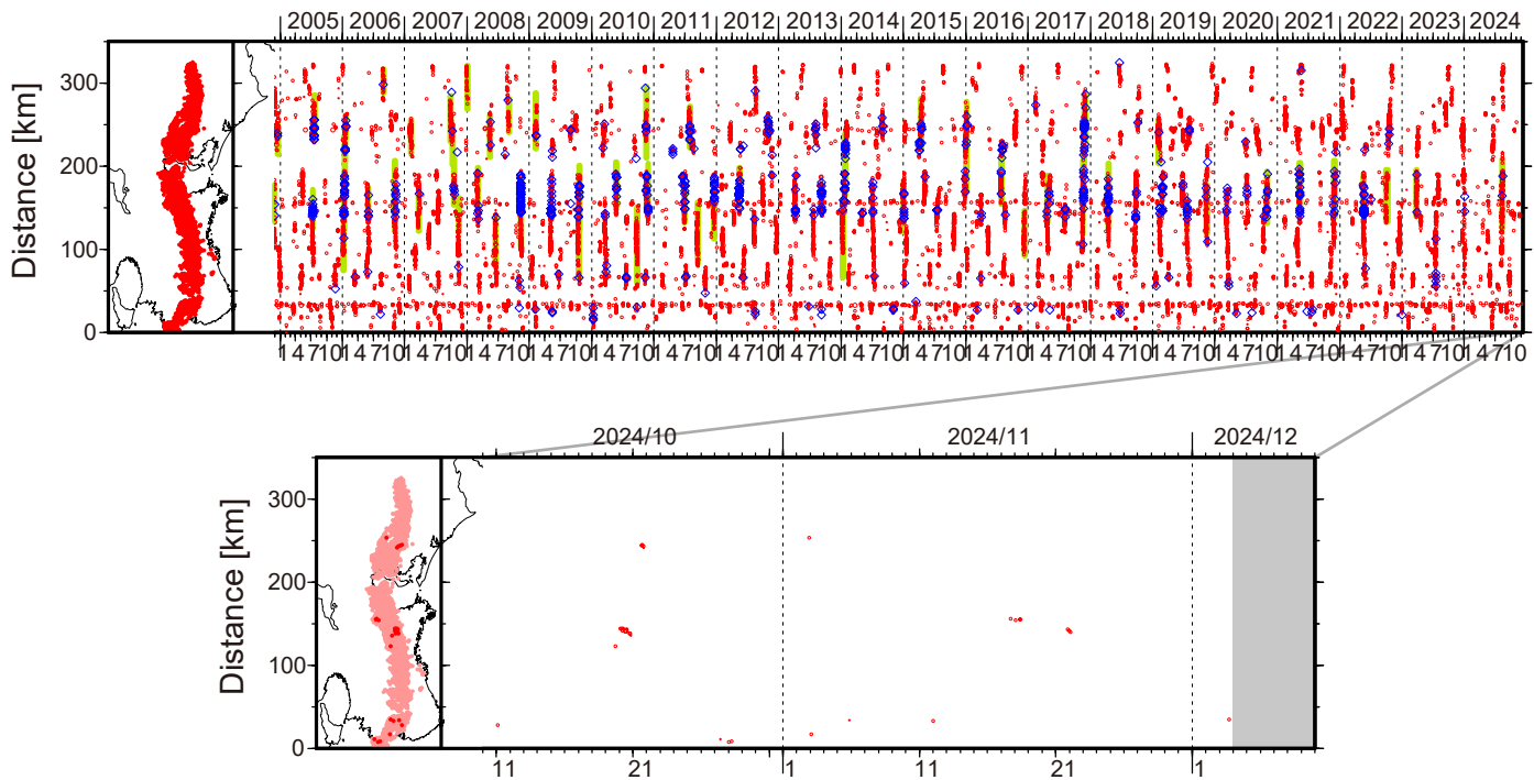
図1. 紀伊半島・東海地域における2004年12月～2024年12月3日までの深部低周波微動の時空間分布（上図）. 赤丸はエンベロープ相関・振幅ハイブリッド法 (Maeda and Obara, 2009) およびクラスタ処理 (Obara et al., 2010) によって1時間毎に自動処理された微動分布の重心である. 青菱形は周期20秒に卓越する超低周波地震 (Ito et al., 2007) である. 黄緑色の太線はこれまでに検出された短期的スロースリップイベント (SSE) を示す. 下図は2024年11月を中心とした期間の拡大図である. 顕著な活動はとくにみられなかったものの、11月17～18日頃には三重県北部において、11月21～22日頃には三重県中部において、それぞれごく小規模な活動がみられた.
