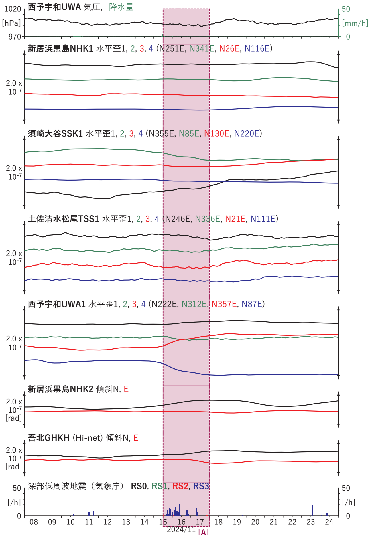
図5 歪・傾斜の時間変化(1) (2024/11/08 00:00-2024/11/25 00:00 (JST))
