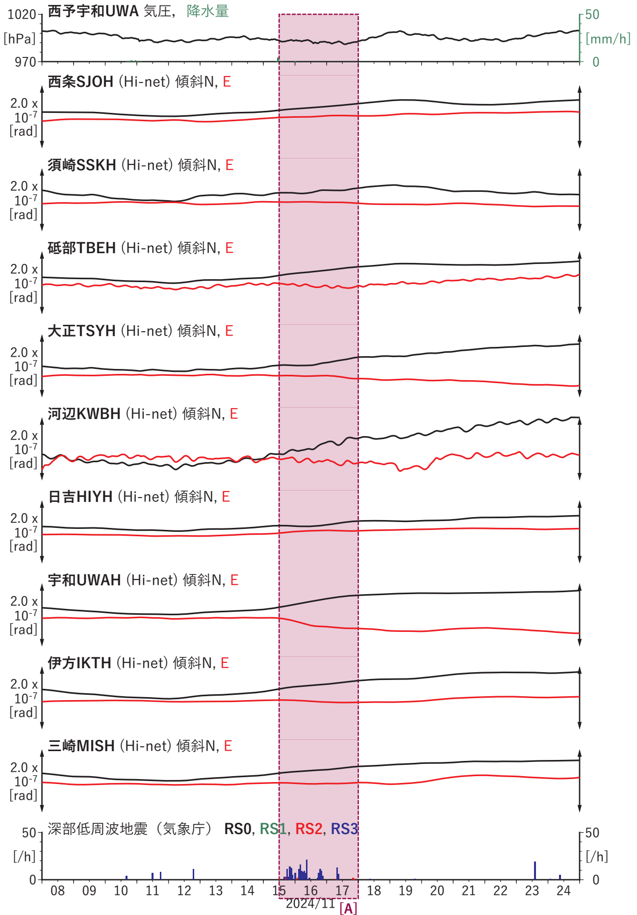
図5 歪・傾斜の時間変化(2) (2024/11/08 00:00-2024/11/25 00:00 (JST))
