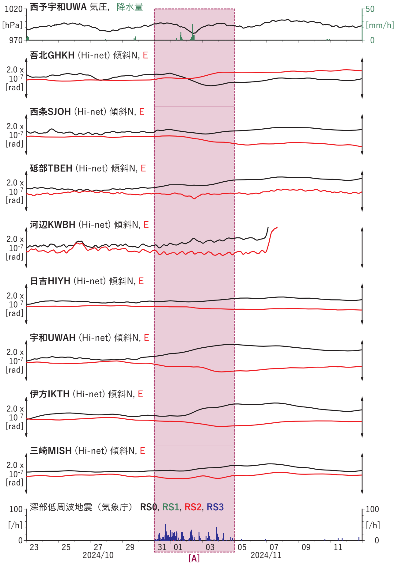
図2 歪・傾斜の時間変化(2) (2024/10/23 00:00-2024/11/13 00:00 (JST))
