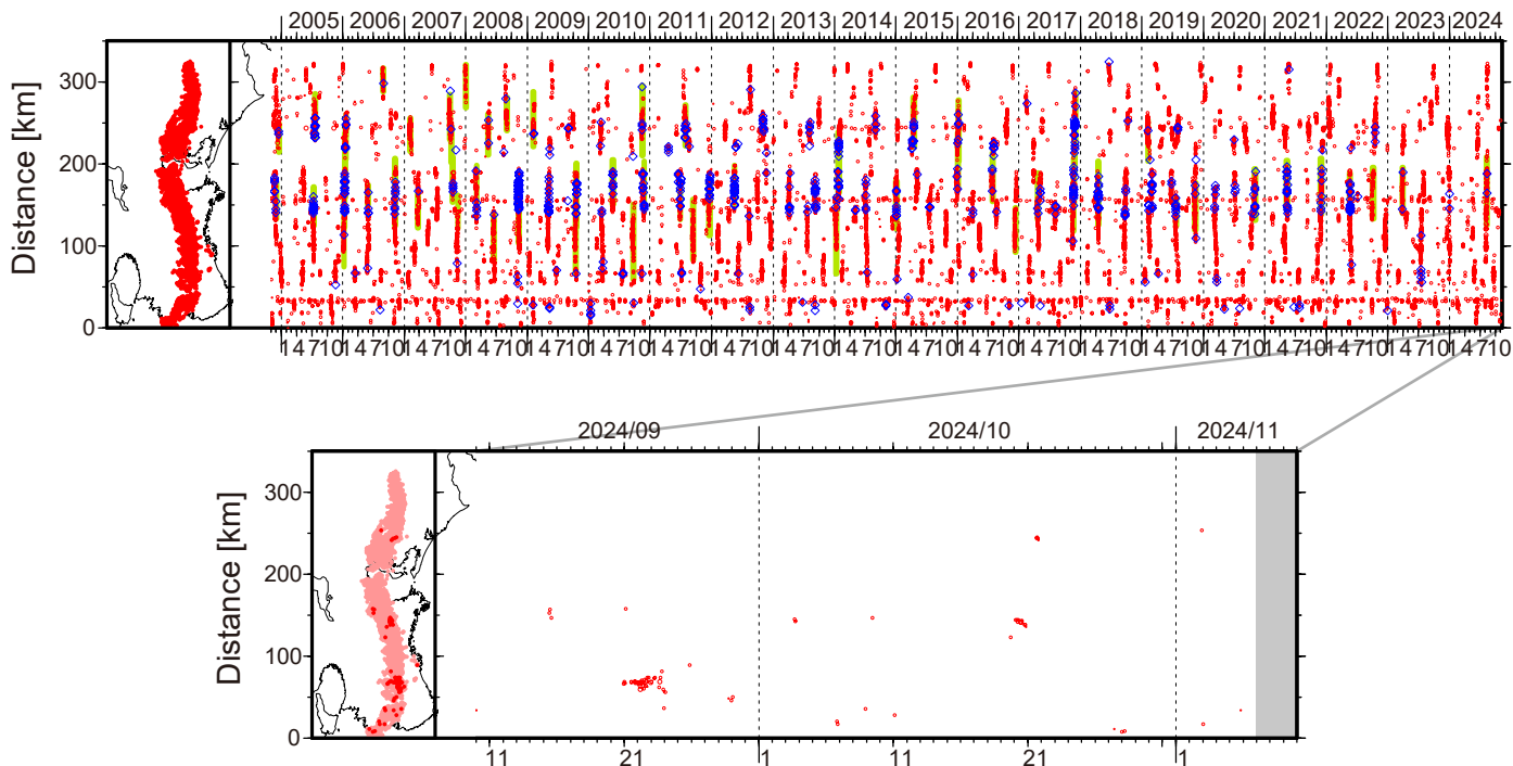
図1. 紀伊半島・東海地域における2004年11月～2024年11月6日までの深部低周波微動の時空間分布(上图). 赤丸はエンベロープ相関・振幅ハイブリッド法(Maeda and Obara, 2009)およびクラスタ処理(Obara et al., 2010)によって1時間毎に自動処理された微動分布の重心である. 青菱形は周期20秒に卓越する超低周波地震(Ito et al., 2007)である. 黄緑色の太線はこれまでに検出された短期的スロースリップイベント(SSE)を示す. 下图は2024年10月を中心とした期間の拡大図である. 顕著な活動はとくにみられなかったものの, 10月19～20日頃には, 三重県中部から三重・奈良県境付近で小規模な微動活動がみられた. 10月3日頃には三重県中部において, 10月21日頃には愛知県中部において, 10月27～28日頃には和歌山県中部において, それぞれごく小規模な活動がみられた.
