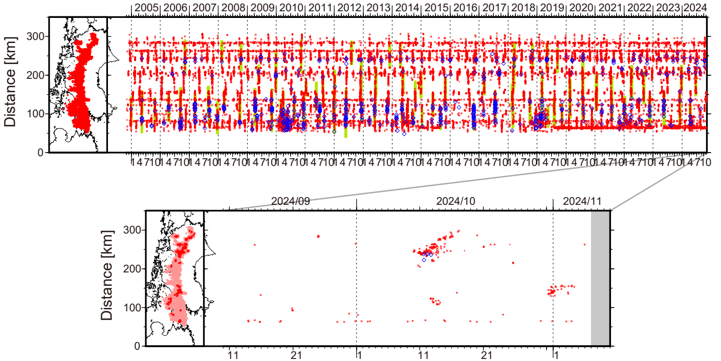
図1. 四国における2004年11月～2024年11月6日までの深部低周波微動の時空間分布(上図). 赤丸はエンベロープ相関・振幅ハイブリッド法(Maeda and Obara, 2009)およびクラスタ処理(Obara et al., 2010)によって1時間毎に自動処理された微動分布の重心である. 青菱形は周期20秒に卓越する超低周波地震(Ito et al., 2007)である. 黄緑色太線は, これまでに検出された短期的スロースリップイベント(SSE)を示す. 下図は2024年10月を中心とした期間の拡大図である. 10月10～18日頃には愛媛県東部から徳島県東部において活発な微動活動がみられた. この活動は愛媛・香川・徳島県境付近で開始したのち東西両方向に拡大し, 13日頃からは主に東方向への活動域の移動がみられた. 10月31日～11月4日頃には愛媛県西部において, やや活発な活動がみられ, 東方向への若干の活動域の移動がみられた. 10月12～14日頃には愛媛県西部において, 小規模な活動がみられた.
