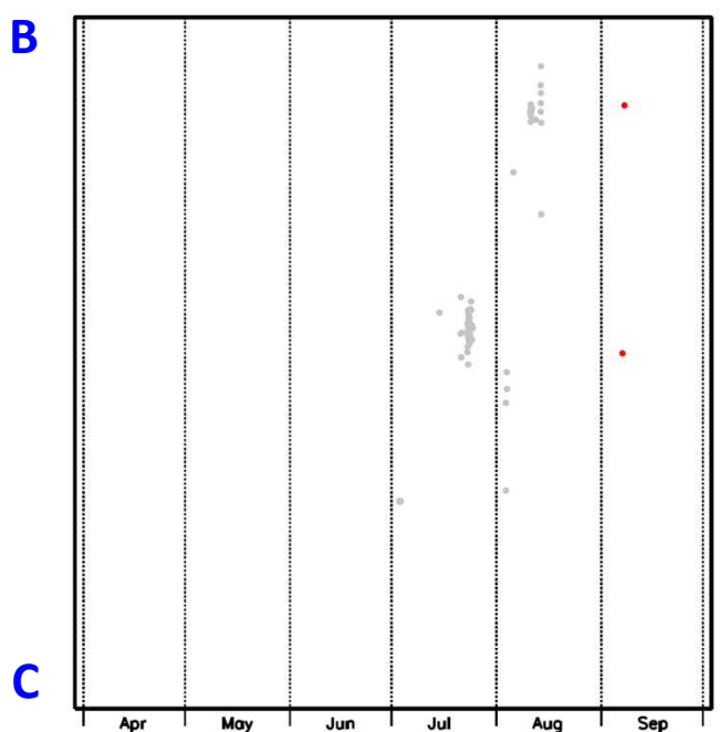
領域a内の時空間分布図(B-C投影) (2024年4月1日～2024年9月30日)
