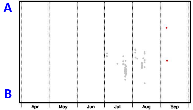
領域a内の時空間分布図(A-B投影) (2024年4月1日～2024年9月30日)
