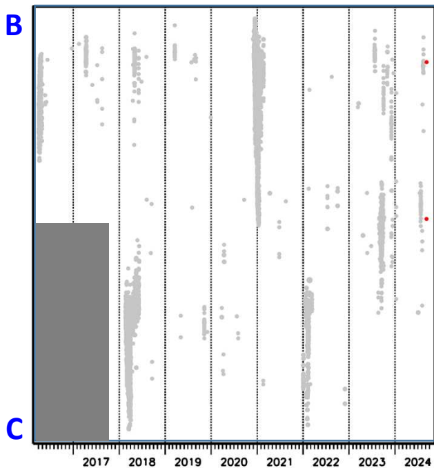
領域a内の時空間分布図(B-C投影) (2016年4月1日～2024年9月30日)
