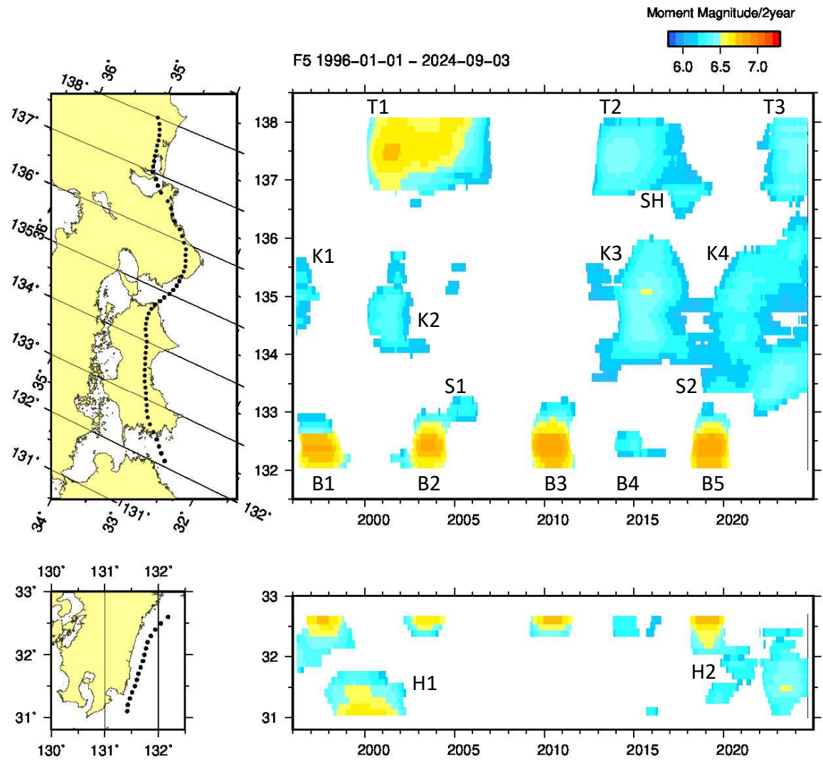
第2図 長期的スロースリップの規模分布 (1996年～2024年9月) 2年間あたりの変化量から推定したモーメントマグニチュード。
