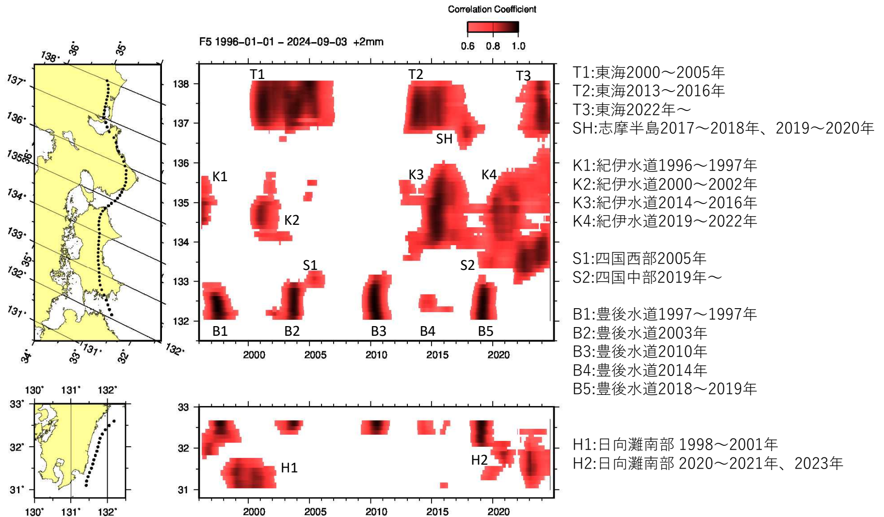
第1図 長期的スロースリップ客観検知図（1996年～2024年9月）
