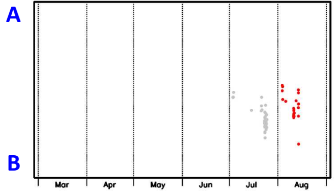
領域a内の時空間分布図(A-B投影) (2024年3月1日～2024年8月31日)
