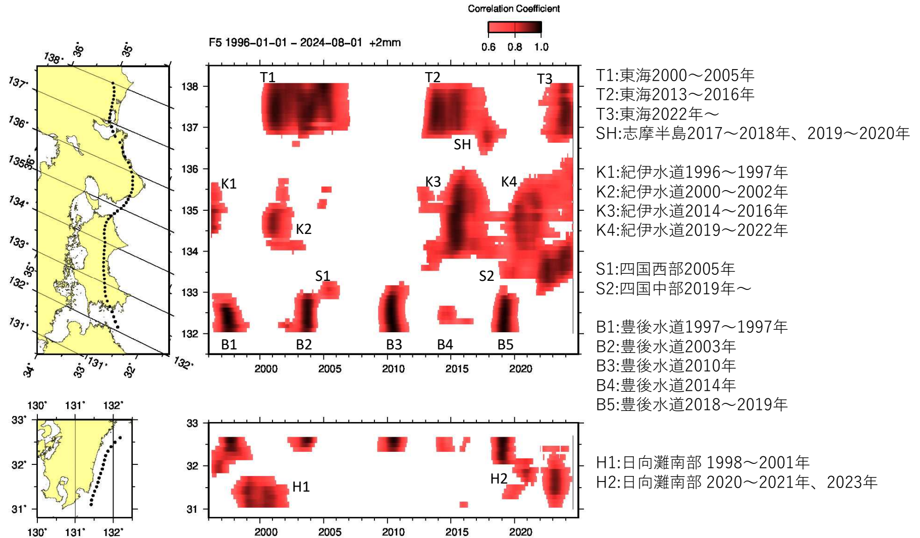
第1図 長期的スロースリップ客観検知図（1996年～2024年8月）
