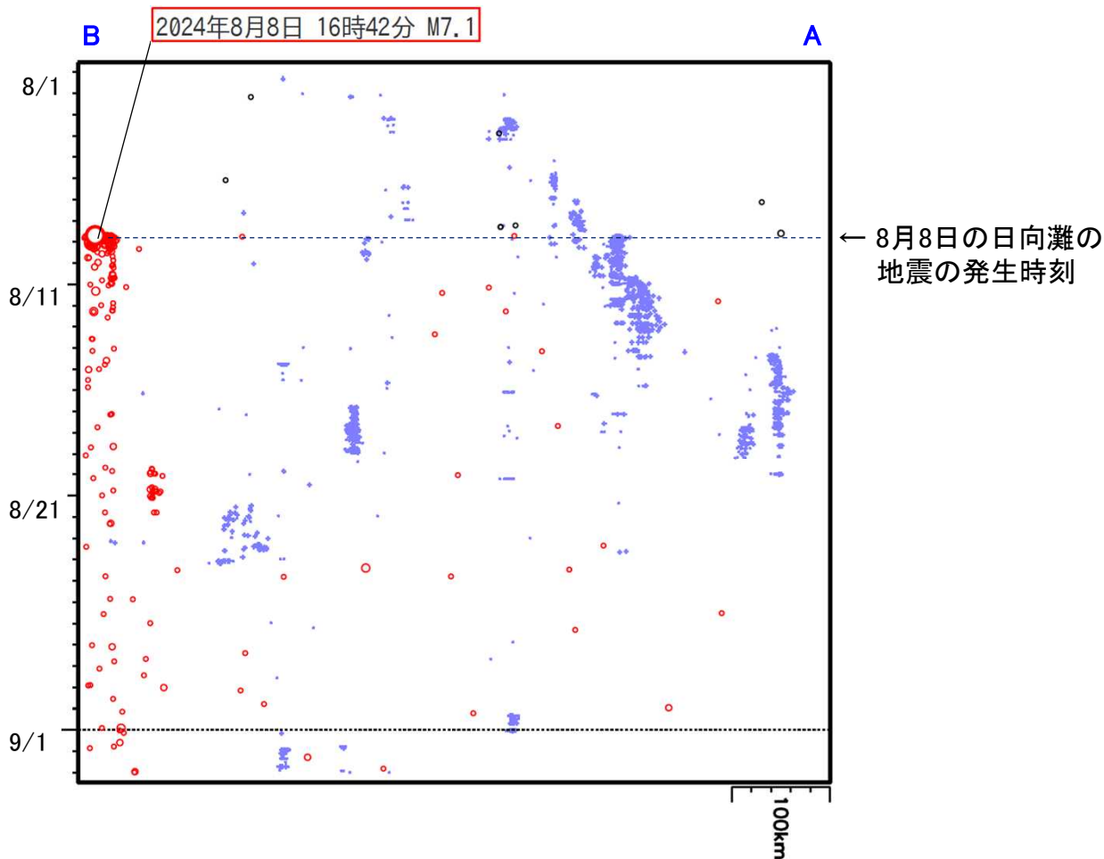
想定震源域内の時空間分布図(A-B投影)
