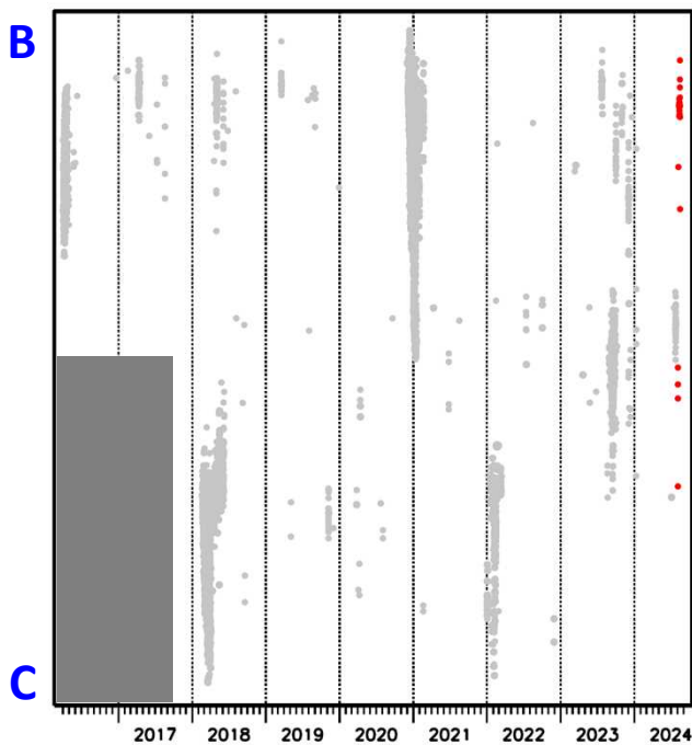
領域a内の時空間分布図(B-C投影) (2016年4月1日～2024年8月31日)
