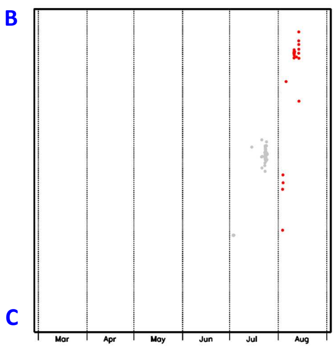
領域a内の時空間分布図(B-C投影) (2024年2月1日～2024年8月31日)
