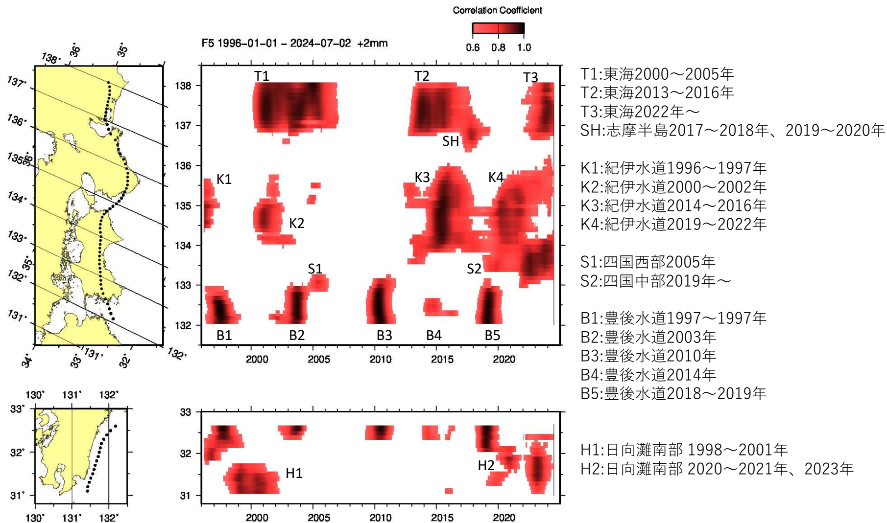
第1図 長期的スロースリップ客観検知図（1996年～2024年7月） スロースリップに伴う非定常変位の範囲（場所、時間）を赤～黒で示す。色が濃いほどスロースリップの発生可能性が高い。右端の縦線は最新データ日を示す。なお、これは変位が検出された範囲で、変動源自体の範囲ではない。
