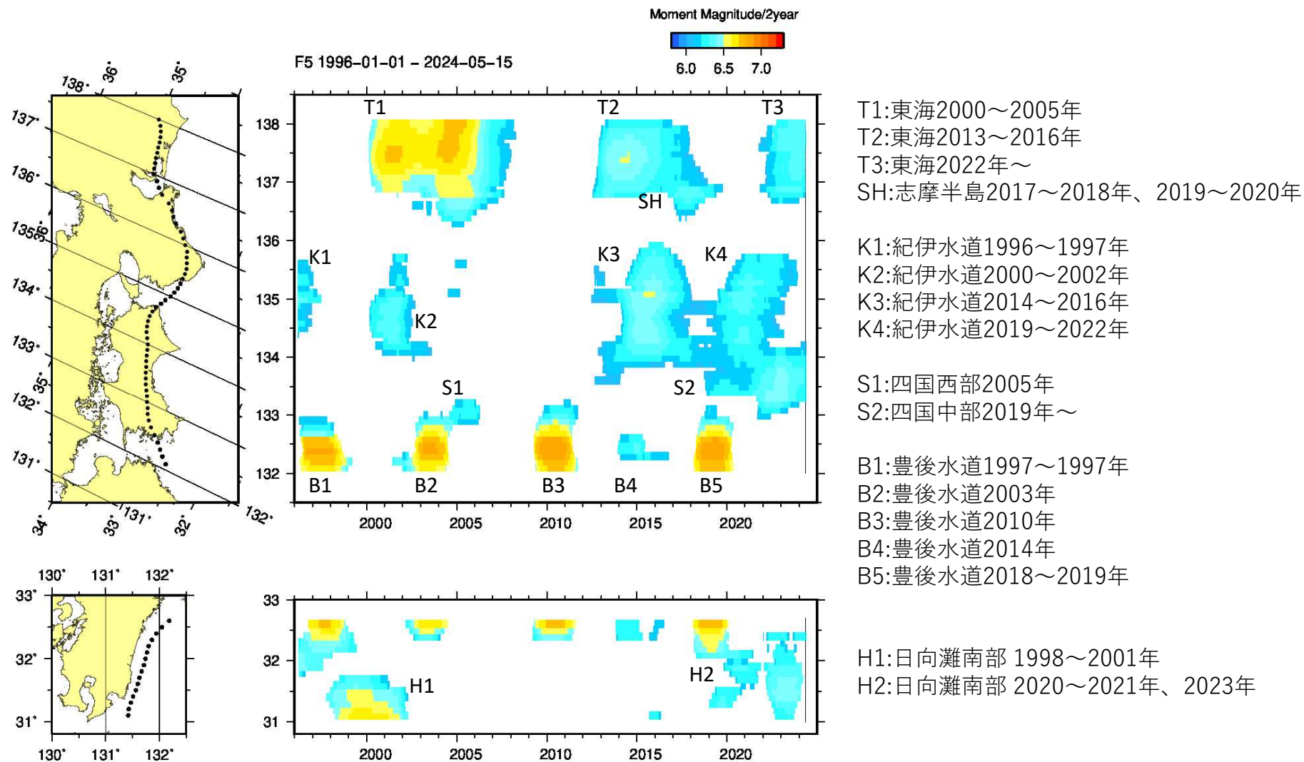
第2図 長期的スロースリップの規模分布（1996年～2024年5月） 2年間あたりの変化量から推定したモーメントマグニチュード。
