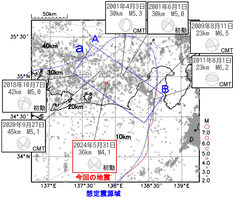
震央分布図 (1997年10月1日～2024年5月31日、 深さ0～80km、 M \geq 2.0 ) 2024年5月31日の地震を赤色で表示
