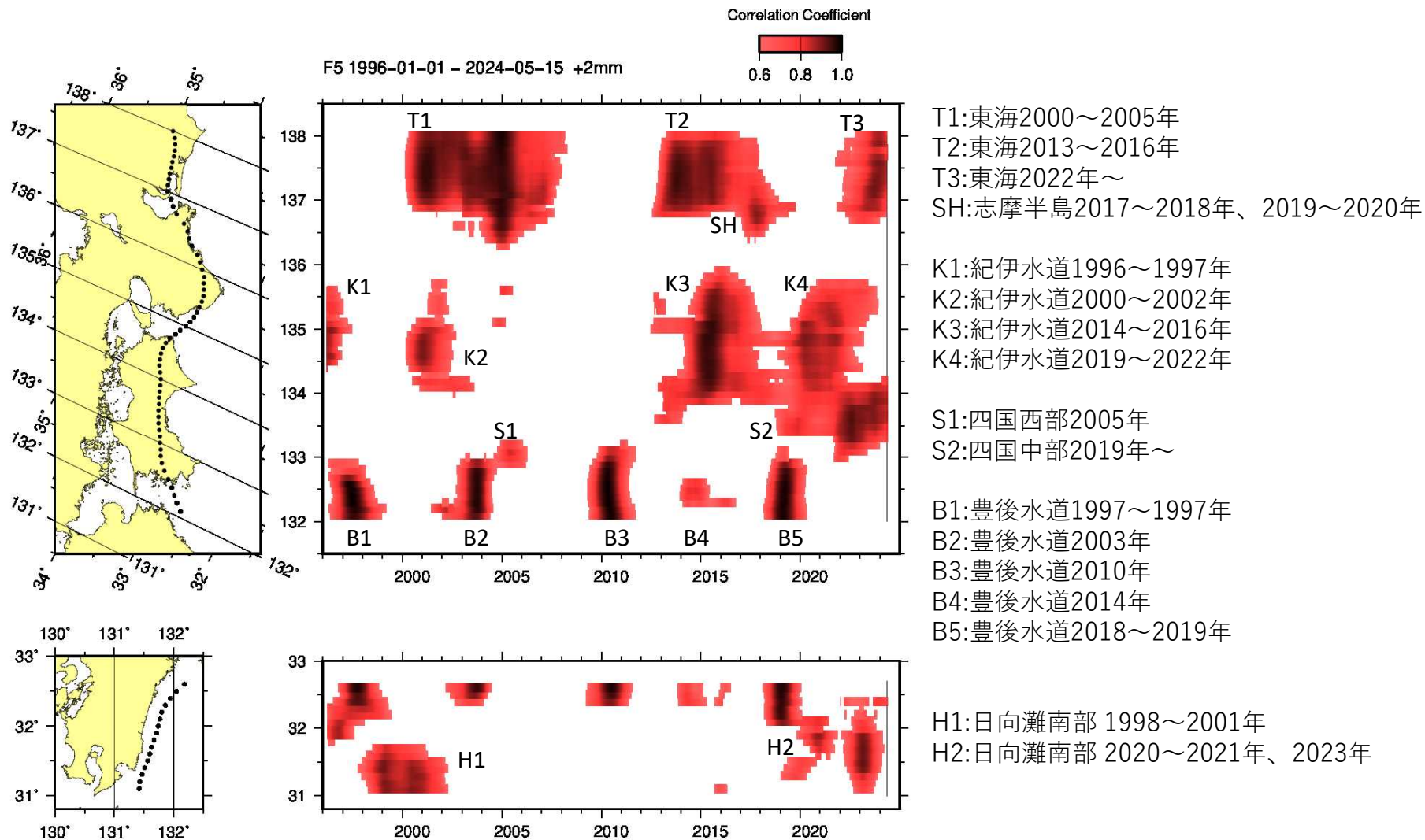
第1図 長期的スロースリップ客観検知図（1996年～2024年5月）
