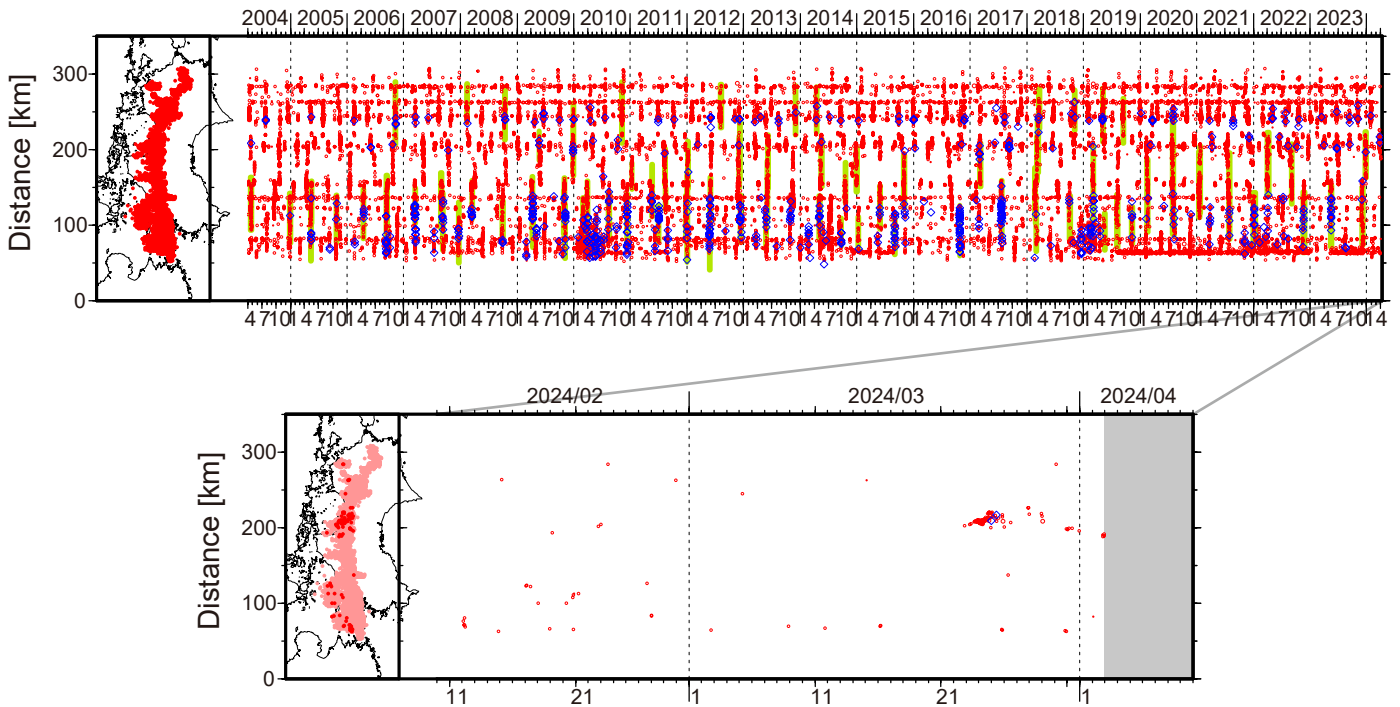
図1. 四国における2004年4月～2024年4月2日までの深部低周波微動の時空間分布(上図). 赤丸はエンベロップ相関・振幅ハイブリッド法(Maeda and Obara, 2009)およびクラスタ処理(Obara et al., 2010)によって1時間毎に自動処理された微動分布の重心である. 青菱形は周期20秒に卓越する超低周波地震(Ito et al., 2007)である. 黄緑色太線は、これまでに検出された短期的スロースリップイベント(SSE)を示す. 下図は2024年3月を中心とした期間の拡大図である. 3月22日頃から愛媛県東部で微動活動が開始している. この活動では、やや東方向への活動域の拡大がみられたのち、26日頃からは活動が散発的となっている.
