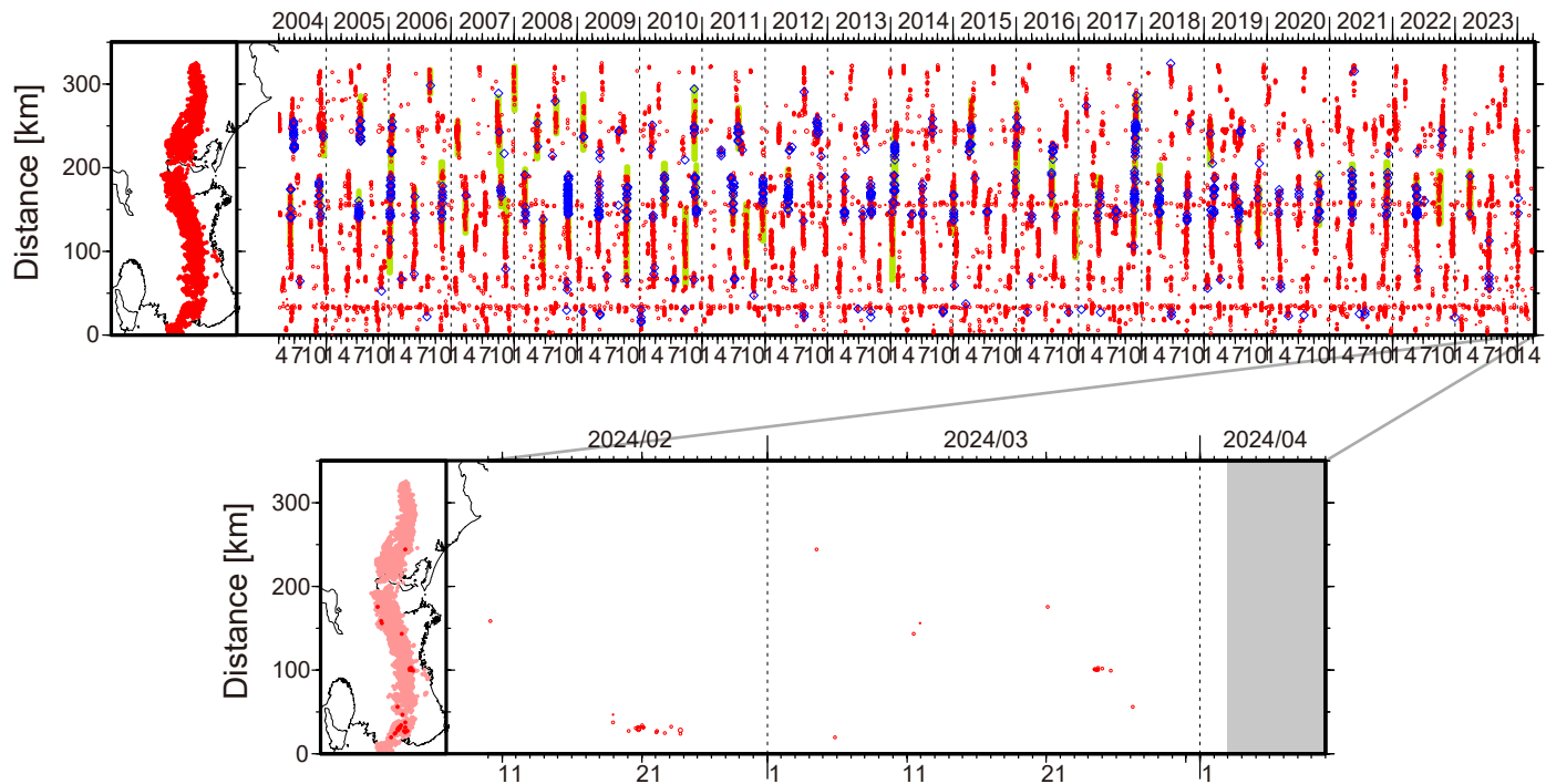
図1. 紀伊半島・東海地域における2004年4月～2024年4月2日までの深部低周波微動の時空間分布（上図）。赤丸はエンベロープ相関・振幅ハイブリッド法 (Maeda and Obara, 2009) およびクラスター処理 (Obara et al., 2010) によって1時間毎に自動処理された微動分布の重心である。青菱形は周期20秒に卓越する超低周波地震 (Ito et al., 2007) である。黄緑色の太線はこれまでに検出された短期的スロースリップイベント (SSE) を示す。下図は2024年3月を中心とした期間の拡大図である。3月以降の期間において、顕著な活動はみられなかったものの、3月24～25日頃に三重・奈良県境付近において、小規模な微動活動がみられた。
