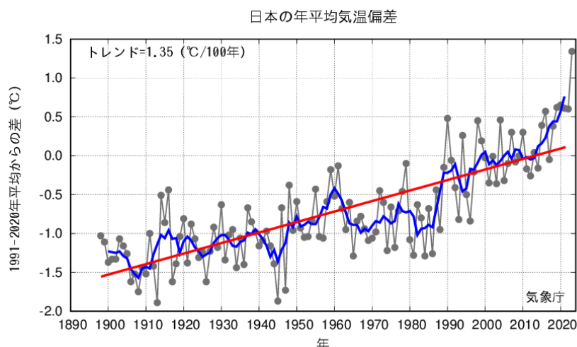
図 1 日本の平均気温偏差（年平均）の経年変化（1898～2023 年、速報）と順位表（上位 10 年）
