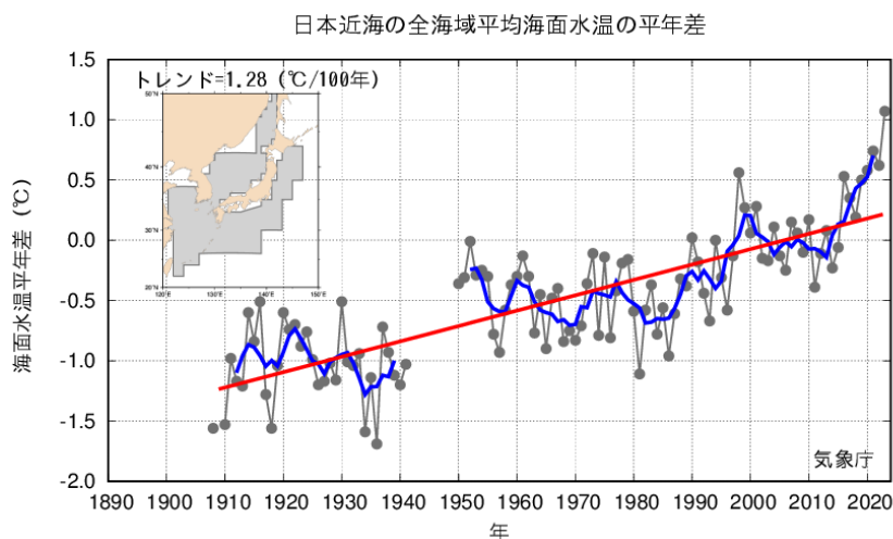
図2 日本近海の全海域平均海面水温（年平均）の平年差の経年変化（1908～2023年、速報）と順位表（上位10位まで）
