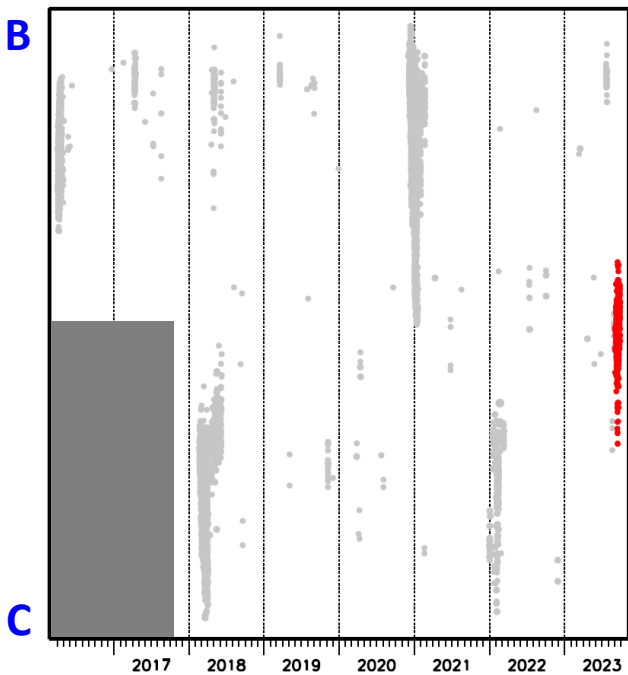
領域a内の時空間分布図(B-C投影) (2016年4月1日～2023年9月30日)
