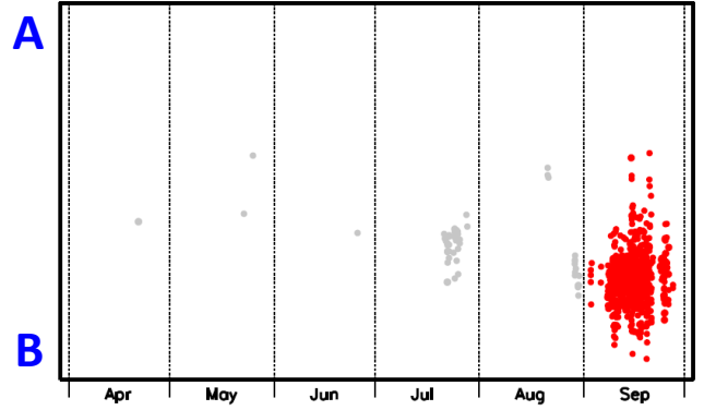
領域a内の時空間分布図(A-B投影) (2023年4月1日～2023年9月30日)
