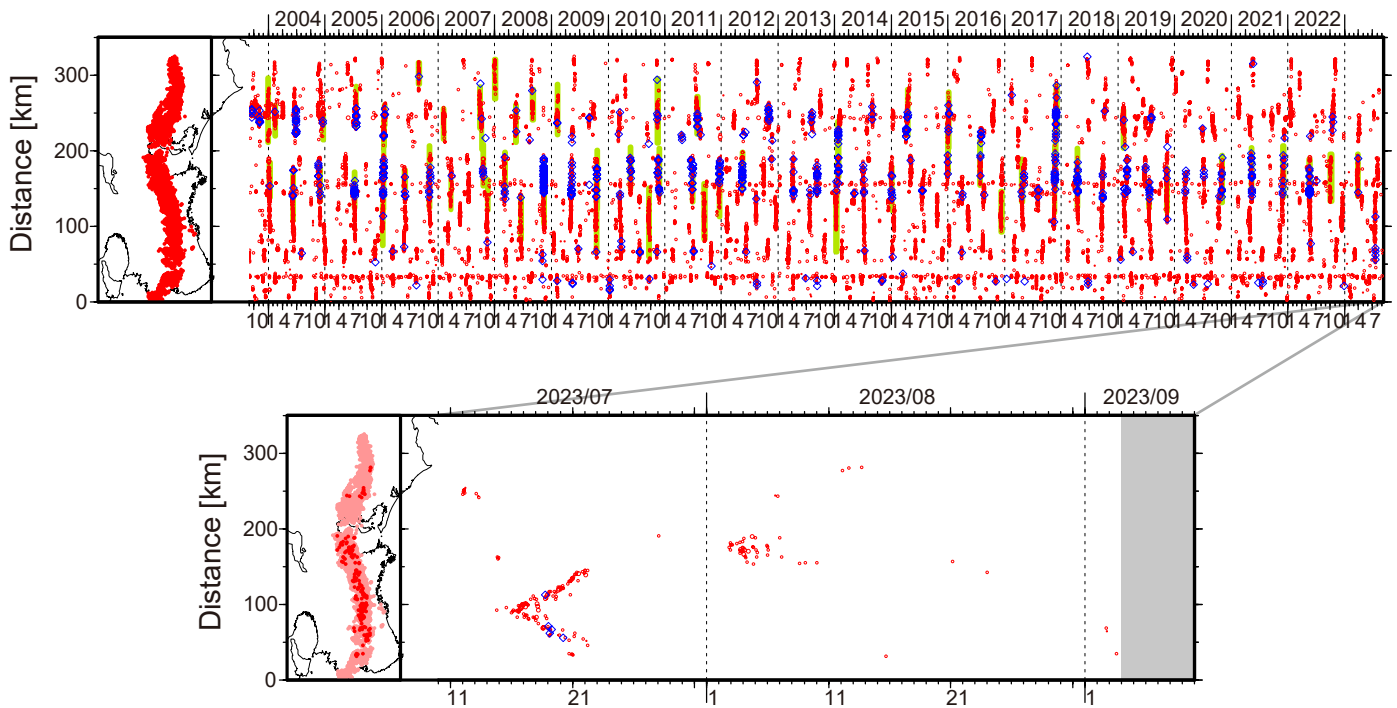
図1. 紀伊半島・東海地域における2003年9月～2023年9月3日までの深部低周波微動の時空間分布(上図). 赤丸はエンベロープ相関・振幅ハイブリッド法(Maeda and Obara, 2009)およびクラスタ処理(Obara et al., 2010)によって1時間毎に自動処理された微動分布の重心である. 青菱形は周期20秒に卓越する超低周波地震(Ito et al., 2007)である. 黄緑色の太線はこれまでに検出された短期的スロースリップイベント(SSE)を示す. 下図は2023年8月を中心とした期間の拡大図である. 8月2～10日頃には三重県北部において、やや活発な活動がみられた. この活動では北東・南西両方向への活動域の拡大がややみられ、その後7日頃から活動は低調となった. 9月2～3日頃には奈良県南部から和歌山県中部において、ごく小規模な微動活動がみられた. 8月12日3:09頃に三河湾付近の深さ約39kmで発生したM4.4の地震(Hi-net暫定値)の後、3:15頃から愛知県東部において微動活動が開始し、クラスタリング処理結果では15時台にも活動が推定されている. 8月23日23:22頃(JST)にアルゼンチン付近の深さ約570kmで発生したM6.2の地震(USGS)の後、8月24日の0:15～0:25頃に三重県中部において微動活動がみられた.
