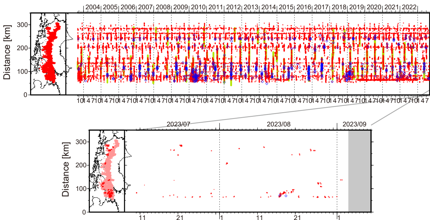
図1. 四国における2003年9月～2023年9月3日までの深部低周波微動の時空間分布(上図). 赤丸はエンベロープ相関・振幅ハイブリッド法(Maeda and Obara, 2009)およびクラスター処理(Obara et al., 2010)によって1時間毎に自動処理された微動分布の重心である. 青菱形は周期20秒に卓越する超低周波地震(Ito et al., 2007)である. 黄緑色太線は、これまでに検出された短期的スロースリップイベント(SSE)を示す. 下図は2023年8月を中心とした期間の拡大図である. 8月16～20日頃には豊後水道においてやや活発な活動がみられた. この活動は豊後水道西部で開始し、やや東方向への活動域の移動がみられた. 8月2～3日頃には愛媛県東部において、8月24～26日頃には香川・徳島県境付近において、それぞれごく小規模な活動がみられた. 8月26～27日頃に愛媛県西部において発生したごく小規模な活動は、8月26日22:29頃に周防灘付近の深さ約74kmで発生したM5.4(Hi-net暫定値)の地震後、22:35頃から開始した.
