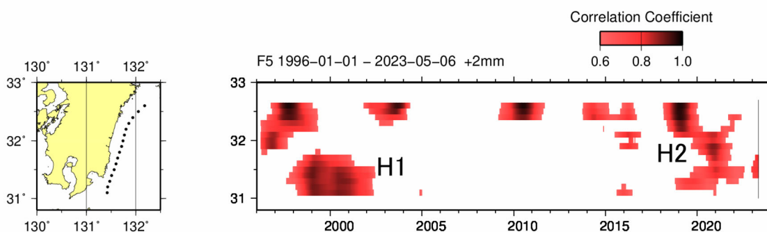
第1図 長期的スロースリップ客観検知図（1996年から2023年5月）
