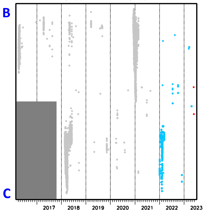
領域a内の時空間分布図(B-C投影) (2016年4月1日～2023年5月31日)
