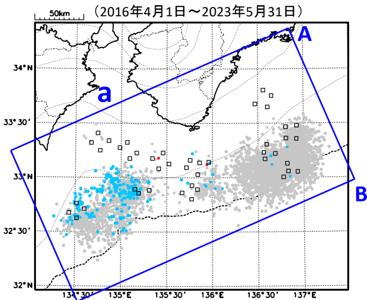
震央分布図
