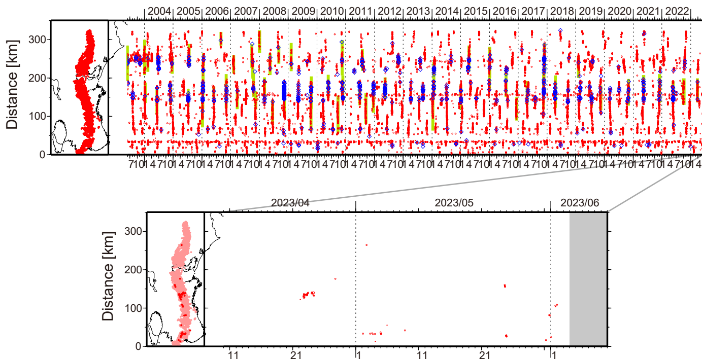
図1. 紀伊半島・東海地域における2003年6月～2023年6月3日までの深部低周波微動の時空間分布(上図). 赤丸はエンベロップ相関・振幅ハイブリッド法 (Maeda and Obara, 2009) およびクラスタ処理 (Obara et al., 2010) によって1時間毎に自動処理された微動分布の重心である. 青菱形は周期20秒に卓越する超低周波地震 (Ito et al., 2007) である. 黄緑色の太線はこれまでに検出された短期的スロースリップイベント (SSE) を示す. 下図は2023年5月を中心とした期間の拡大図である. この期間に顕著な活動はとくにみられなかったものの, 5月3～5日頃および5月24～25日頃には和歌山県中部において, 5月31日～6月2日頃には, 奈良県南部から奈良・三重県境付近において, それぞれごく小規模な活動がみられた.
