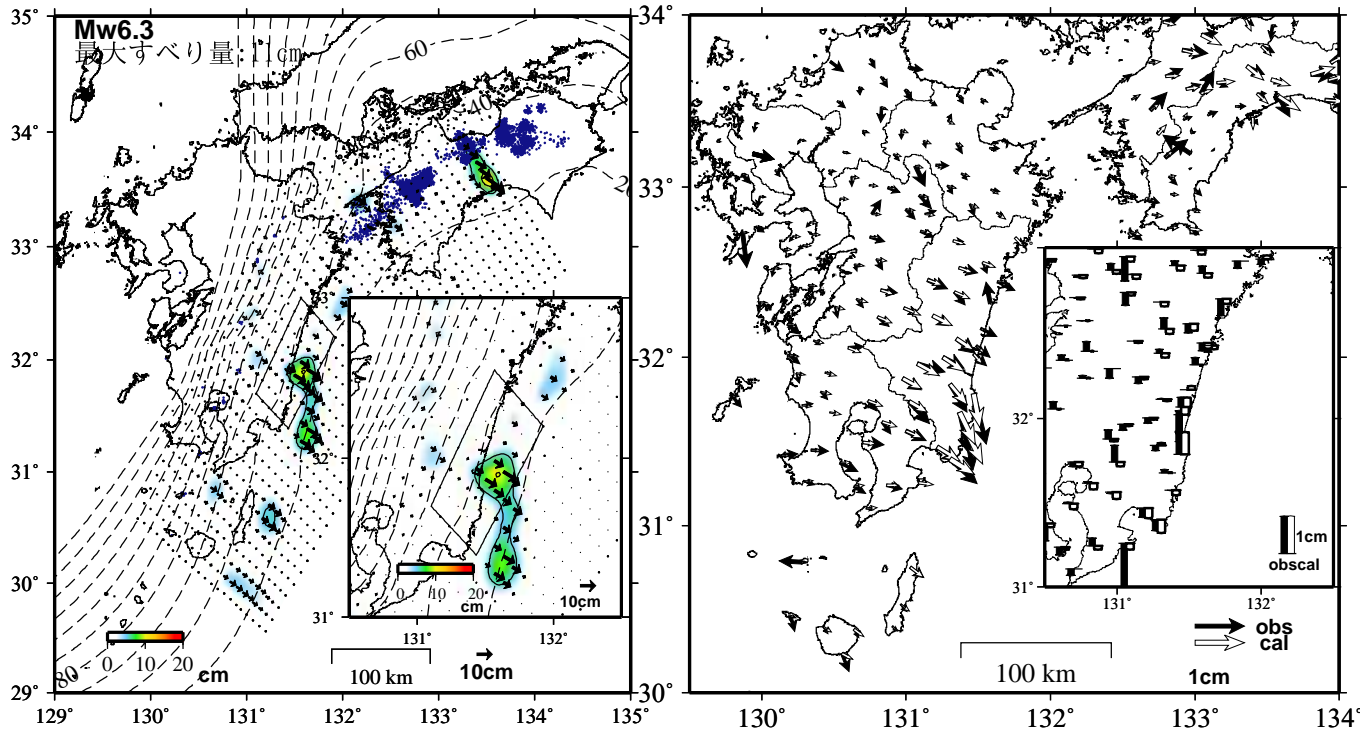
推定すべり分布 (2022/7/1-2023/5/9)
