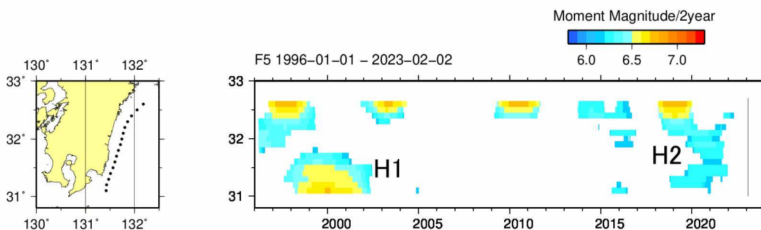
第2図 長期的スロースリップの規模分布（1996年から2023年2月） 2年間あたりの変化量から推定したモーメントマグニチュード。地域略号は第1図と同じ。
