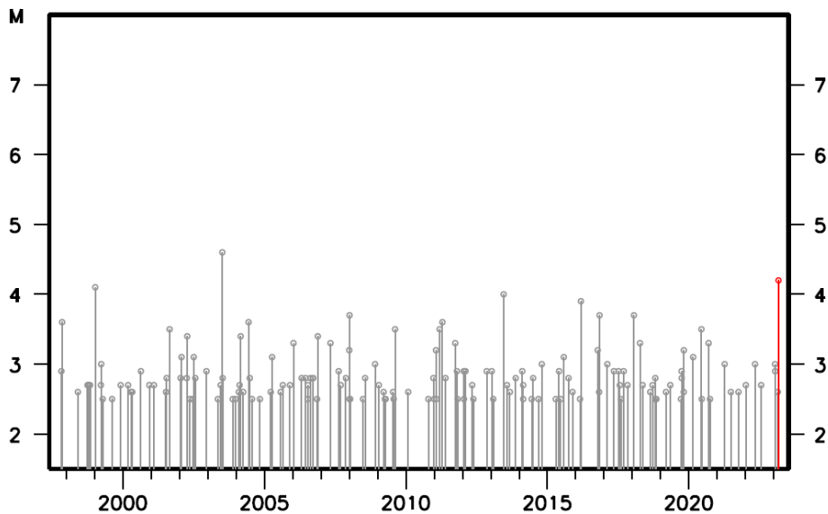
領域 a 内の M-T 図
