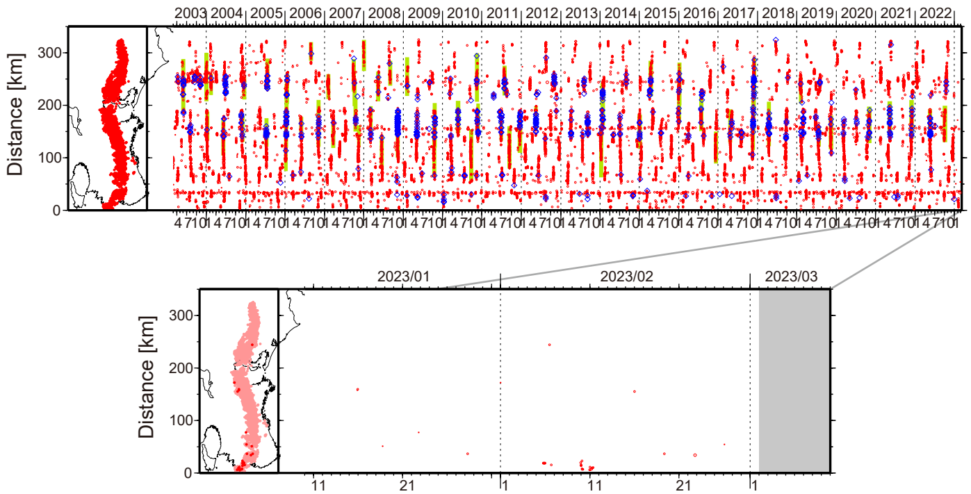
図1. 紀伊半島・東海地域における2003年3月～2023年3月1日までの深部低周波微動の時空間分布(上図). 赤丸はエンベロープ相関・振幅ハイブリッド法(Maeda and Obara, 2009)およびクラスター処理(Obara et al., 2010)によって1時間毎に自動処理された微動分布の重心である. 青菱形は周期20秒に卓越する超低周波地震(Ito et al., 2007)である. 黄緑色の太線はこれまでに検出された短期的スロースリップイベント(SSE)を示す. 下図は2023年2月を中心とした期間の拡大図である. 2月以降の期間において、顕著な活動はとくにみられなかったものの、和歌山県中部において、2月5～6日頃にはごく小規模な活動が、2月9～11日頃には小規模な活動がそれぞれみられた. 2月6日10:17(JST)頃にトルコで発生したMw7.8(USGS)の地震後11:00～11:25頃に、愛知県中部において微動活動がみられ、クラスタリング処理結果においても微動源位置が推定されている(図2).
