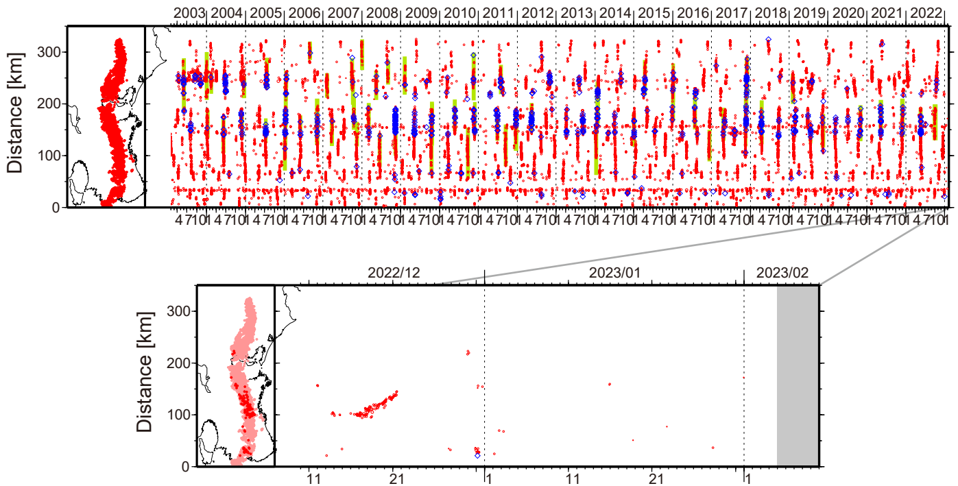
図1. 紀伊半島・東海地域における2003年2月～2023年2月4日までの深部低周波微動の時空間分布(上図). 赤丸はエンベロープ相関・振幅ハイブリッド法(Maeda and Obara, 2009)およびクラスター処理(Obara et al., 2010)によって1時間毎に自動処理された微動分布の重心である. 青菱形は周期20秒に卓越する超低周波地震(Ito et al., 2007)である. 黄緑色の太線はこれまでに検出された短期的スロースリップイベント(SSE)を示す. 下図は2023年1月を中心とした期間の拡大図である. 1月以降の期間において、顕著な活動はとくにみられなかった。
