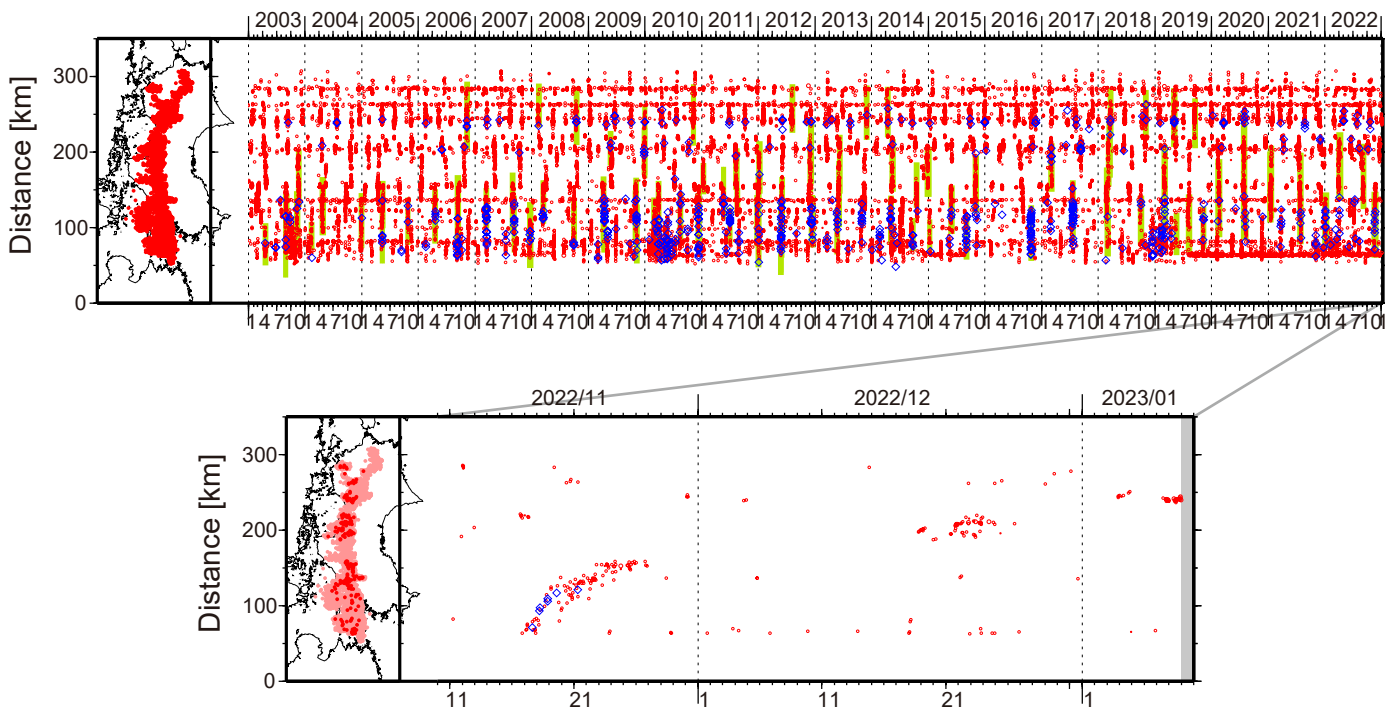
図1. 四国における2003年1月～2023年1月8日までの深部低周波微動の時空間分布(上図). 赤丸はエンベロープ相関・振幅ハイブリッド法(Maeda and Obara, 2009)およびクラスタ処理(Obara et al., 2010)によって1時間毎に自動処理された微動分布の重心である. 青菱形は周期20秒に卓越する超低周波地震(Ito et al., 2007)である. 黄緑色太線は、これまでに検出された短期的スロースリップイベント(SSE)を示す. 下図は2022年12月を中心とした期間の拡大図である. 12月21～26日頃には愛媛県東部において、やや活発な活動がみられた. この活動に先だち、12月18～20日頃には同領域のやや北側において、小規模な活動がみられた. 1月3～4日頃には愛媛・香川・徳島県境付近において、ごく小規模な活動がみられた. 1月7日頃からは、同地域において活動が開始している.
