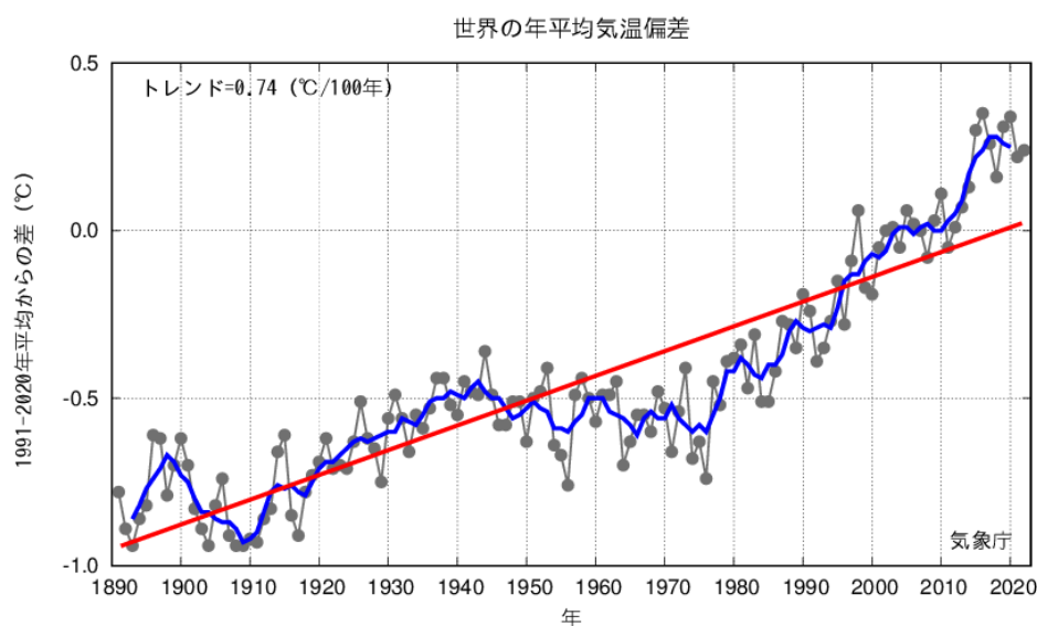
図 1 世界の年平均気温偏差の経年変化（1891～2022 年、速報）
