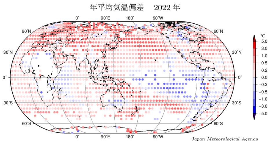
図 2 2022 年の年平均気温偏差の分布図（速報）
