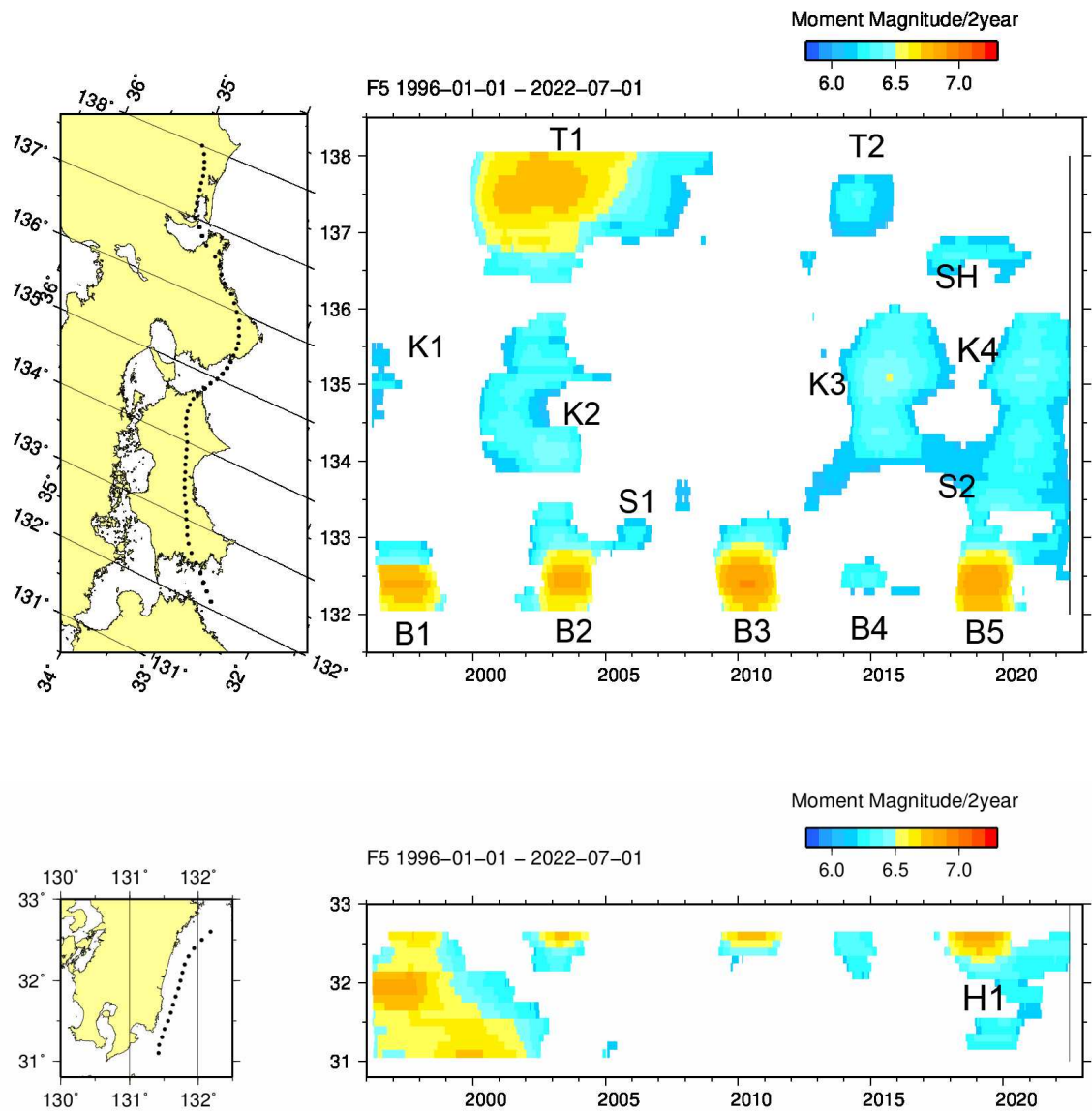
第2図 長期的スロースリップの規模分布（1996年から2022年7月） 2年間あたりの変化量から推定したモーメントマグニチュード。地域略号は第1図と同じ。
