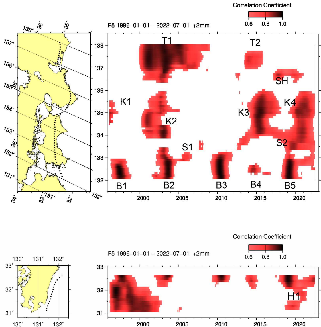
第1図 長期的スロースリップ客観検知図（1996年から2022年7月）
