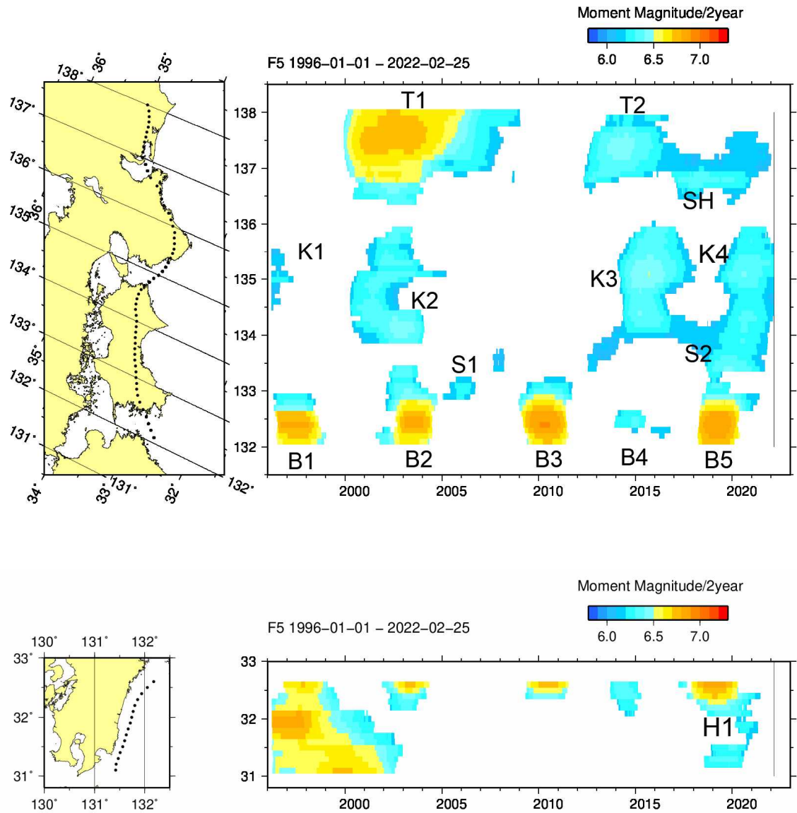
第2図 長期的スロースリップの規模分布（1996年から2022年2月） 2年間あたりの変化量から推定したモーメントマグニチュード。地域略号は第1図と同じ。
