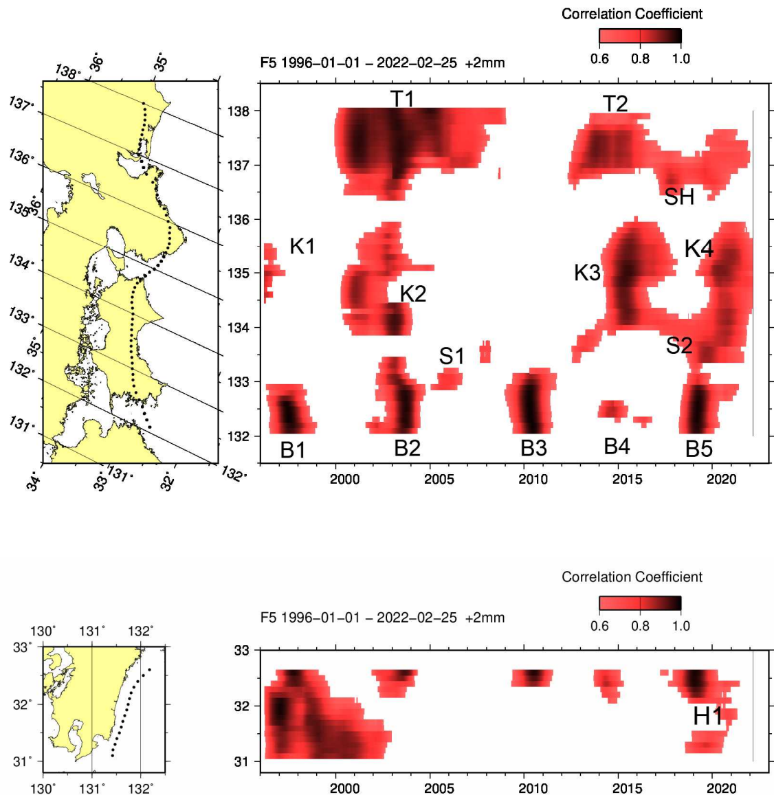
第1図 長期的スロースリップ客観検知図（1996年から2022年2月）
