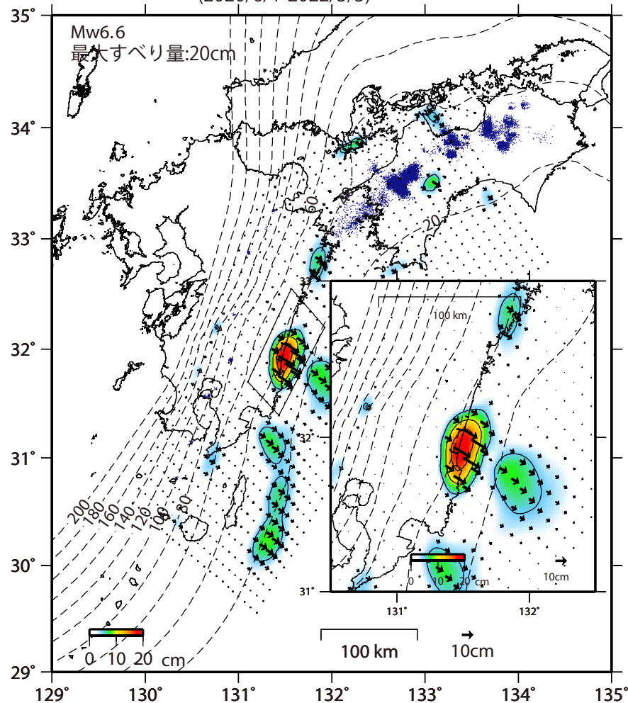
推定すべり分布 (2020/6/1-2022/3/3)
