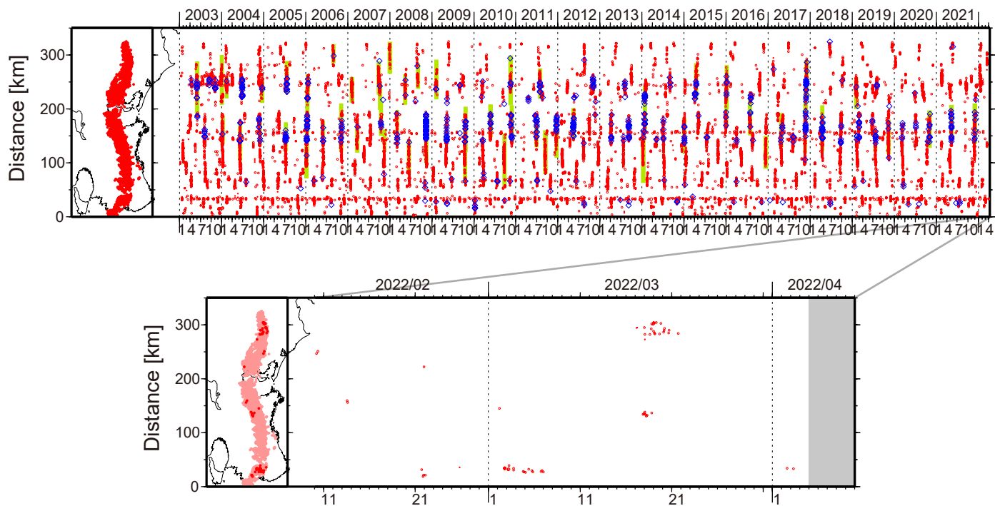
図1. 紀伊半島・東海地域における2003年1月～2022年4月4日までの深部低周波微動の時空間分布(上图). 赤丸はエンベロープ相関・振幅ハイブリッド法(Maeda and Obara, 2009)およびクラスター処理(Obara et al., 2010)によって1時間毎に自動処理された微動分布の重心である. 青菱形は周期20秒に卓越する超低周波地震(Ito et al., 2007)である. 黄緑色の太線はこれまでに検出された短期的スロースリップイベント(SSE)を示す. 下图は2022年3月を中心とした期間の拡大図である. 3月17～21日頃には長野・愛知県境付近から長野県南部において、やや活発な活動がみられた. 3月2～3日頃および3月4～5日頃には、ともに和歌山県中部において、小規模な活動がみられた. 3月17～18日頃には三重・奈良県境付近において、ごく小規模な活動がみられた.
