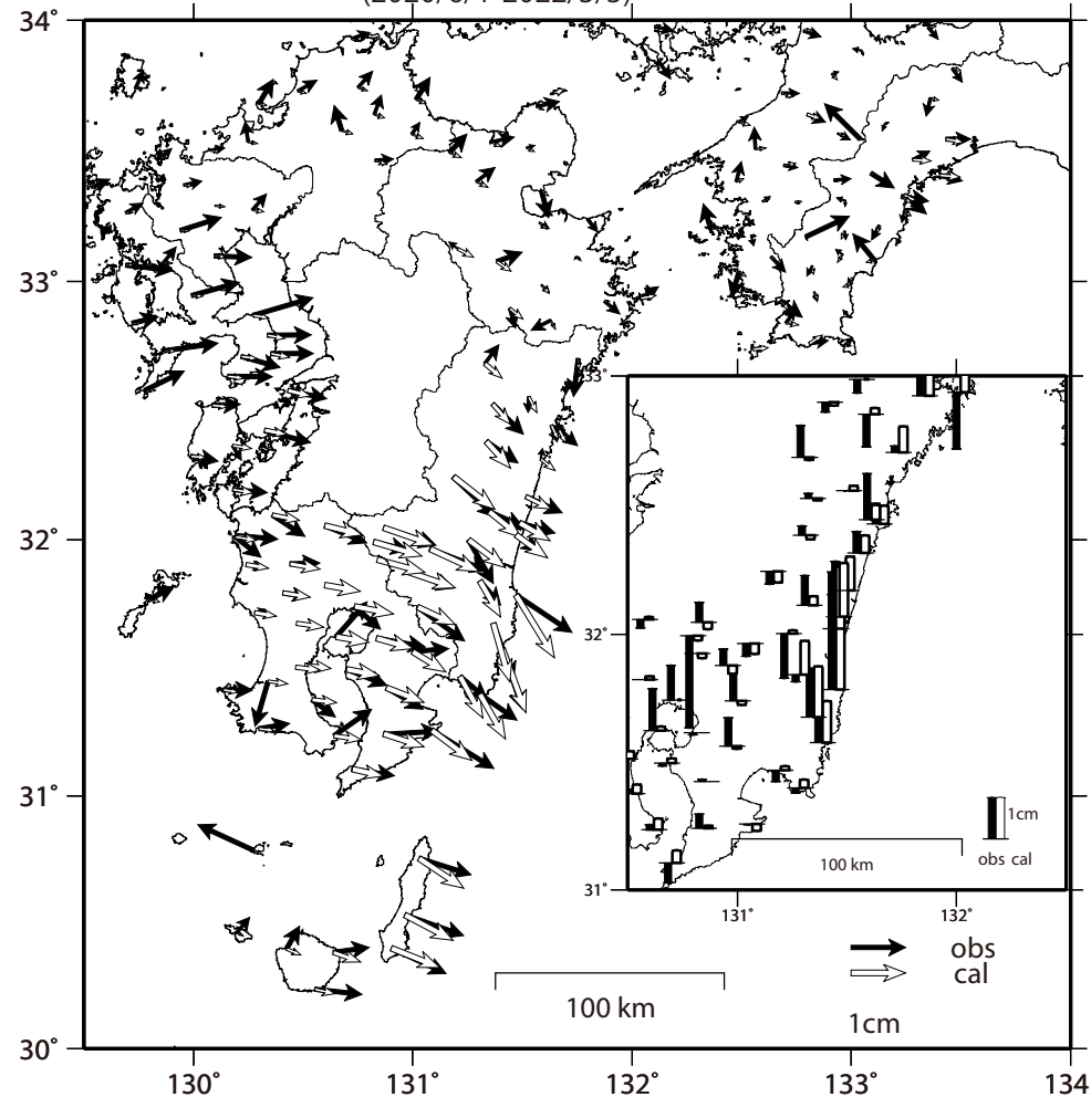
観測値 (黒) と計算値 (白) の比較 (2020/6/1-2022/3/3)
