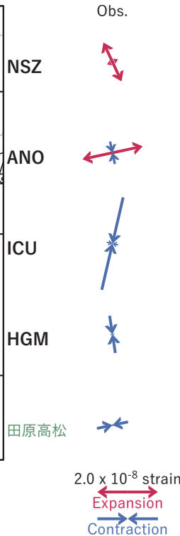
図3 2021/11/27-30の歪・傾斜・水位変化 (図2[A]) を説明する断層モデル。
