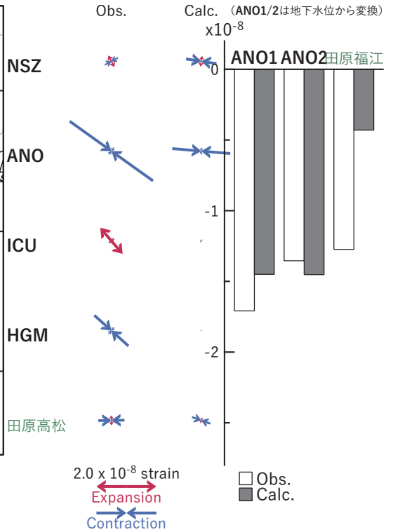
図4 2021/12/01-02の歪・傾斜・水位変化（図2[B]）を説明する断層モデル。
