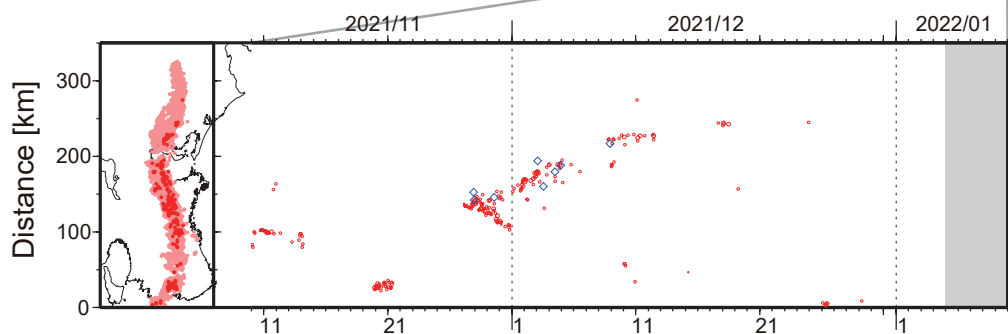
図1. 紀伊半島・東海地域における2003年1月～2022年1月4日までの深部低周波微動の時空間分布(上図). 赤丸はエンベロープ相関・振幅ハイブリッド法 (Maeda and Obara, 2009) およびクラスタ処理 (Obara et al., 2010) によって1時間毎に自動処理された微動分布の重心である. 青菱形は周期20秒に卓越する超低周波地震 (Ito et al., 2007) である. 黄緑色の太線はこれまでに検出された短期的スロースリップイベント (SSE) を示す. 下図は2021年12月を中心とした期間の拡大図である.
