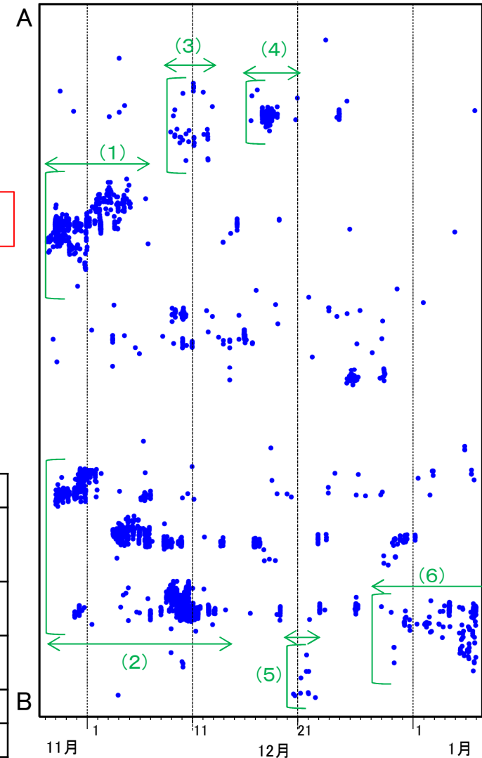
領域a(点線矩形)内の深部低周波地震(微動)の時空間分布図(A-B投影)
