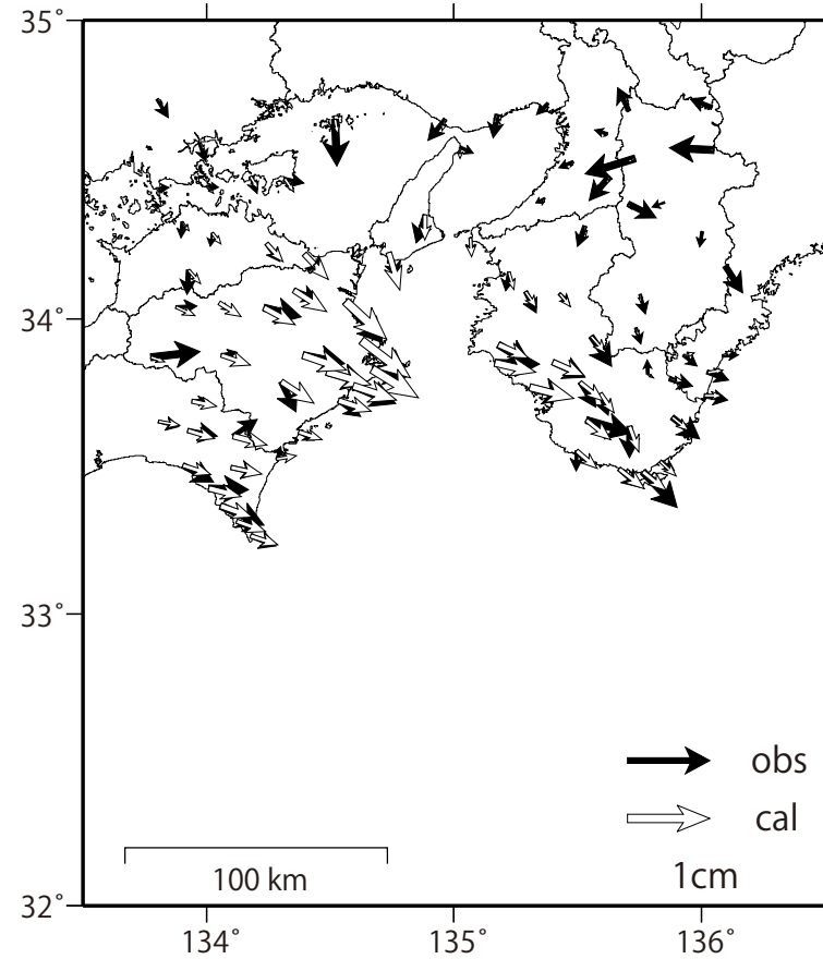
観測値（黒）と計算値（白）の比較 (2020/6/1-2021/12/9)
