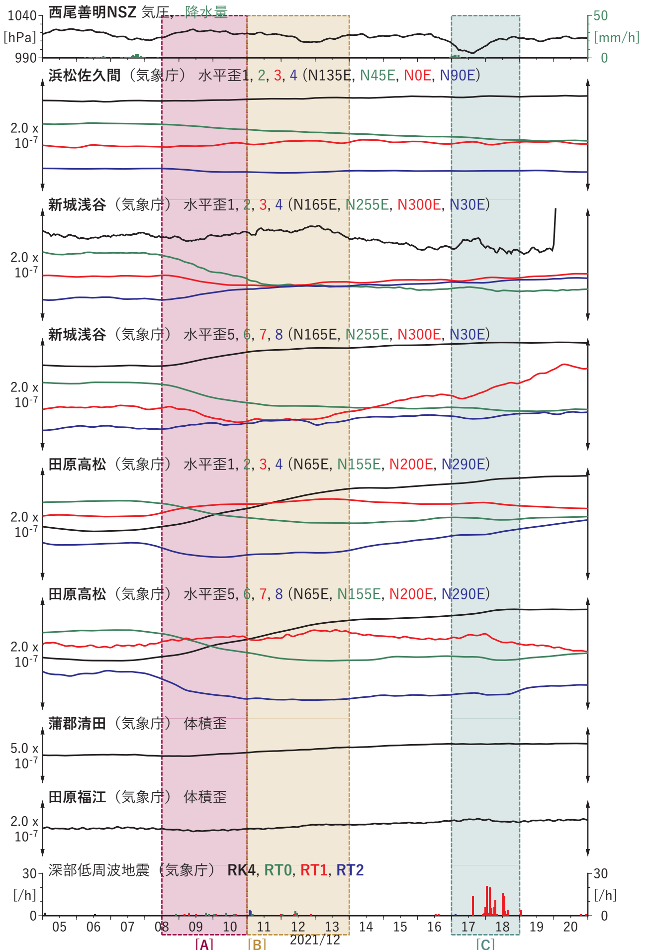
図7 歪・傾斜の時間変化(2) (2021/12/05 00:00-2021/12/21 00:00 (JST))
