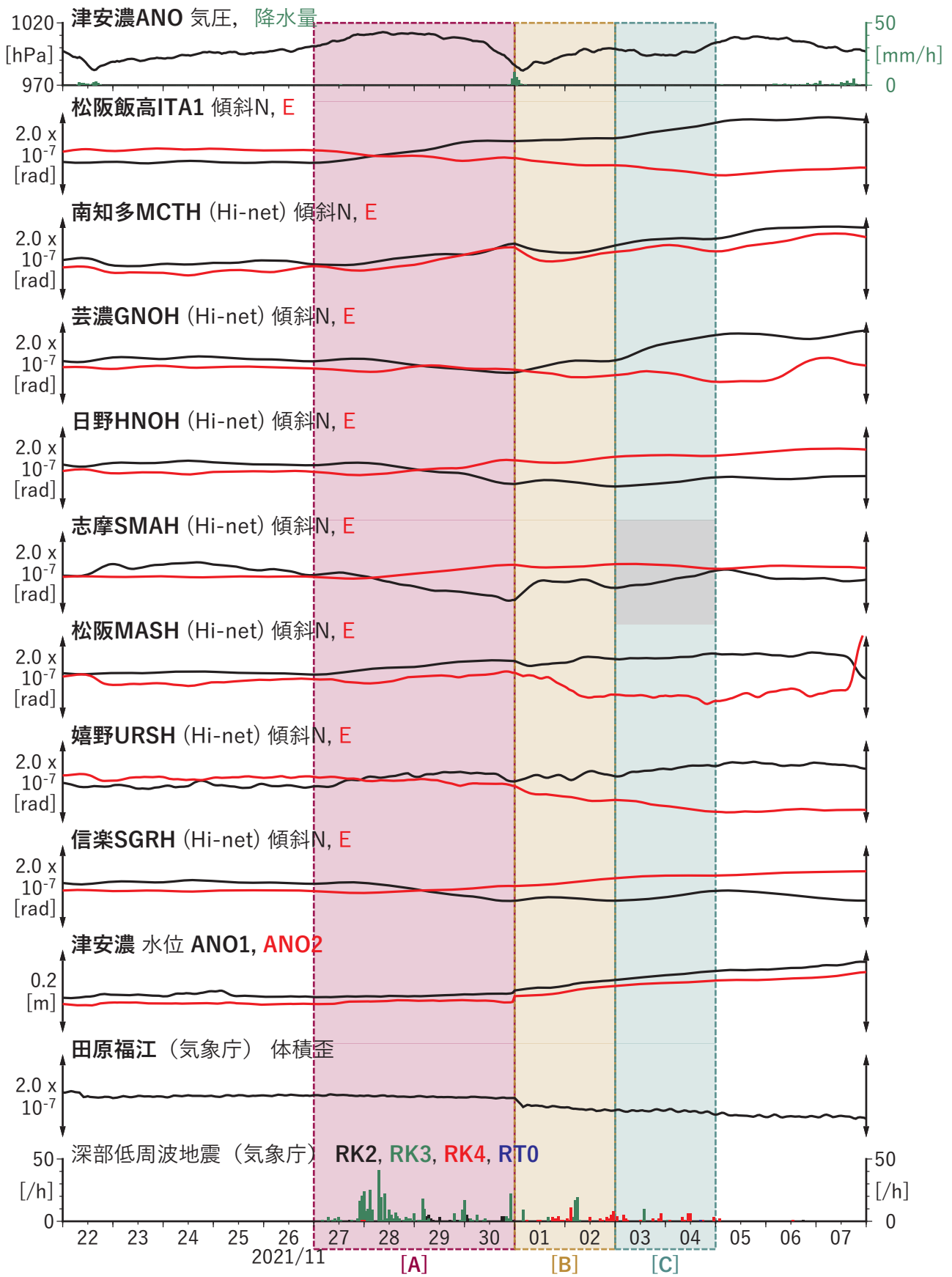
図2 歪・傾斜・水位の時間変化(1) (2021/11/22 00:00-2021/12/08 00:00 (JST))
