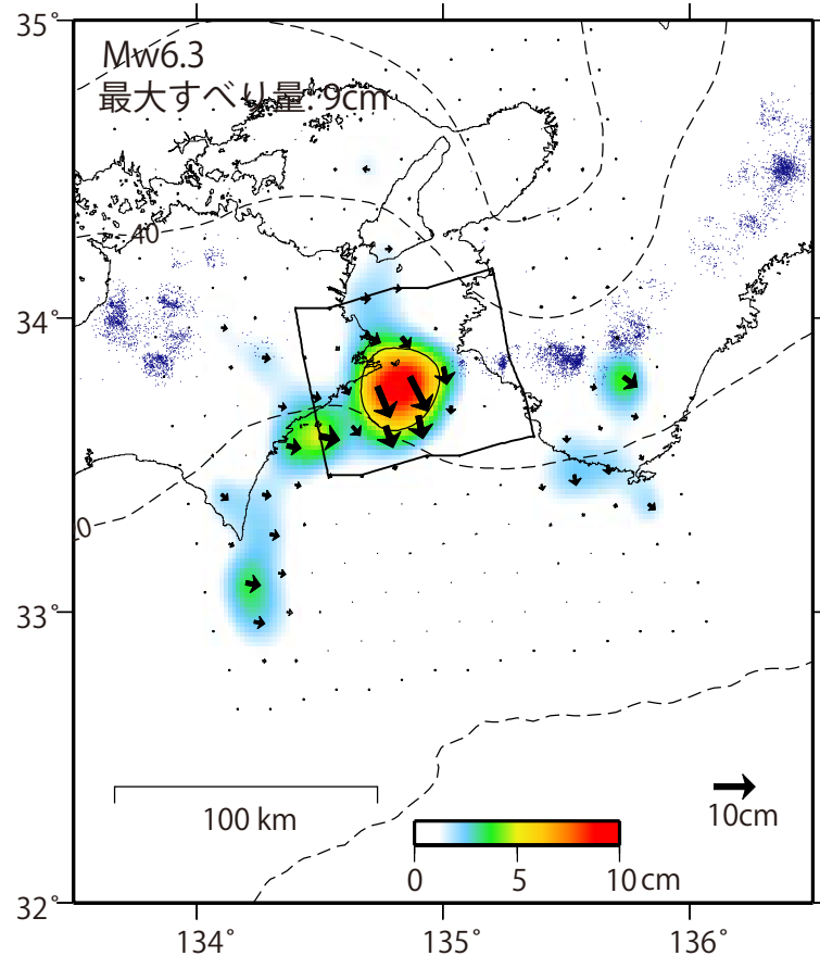
推定すべり分布 (2020/6/1-2021/12/9)
