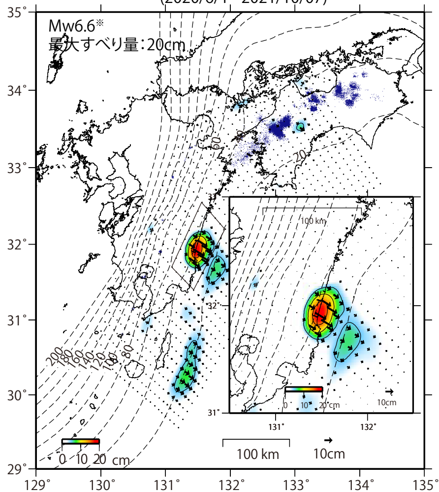
推定すべり分布 (2020/6/1 - 2021/10/7)
