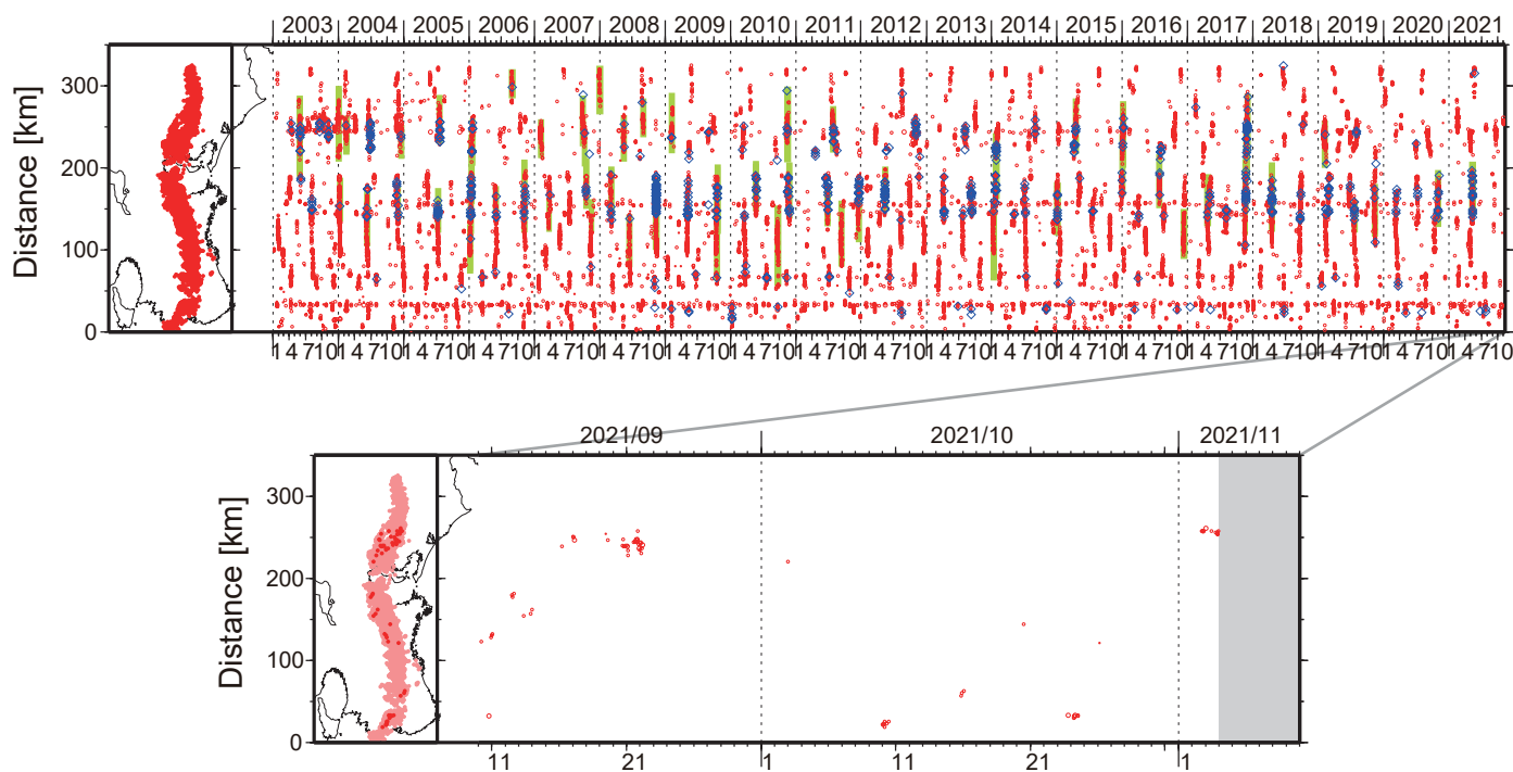
図1. 紀伊半島・東海地域における2003年1月～2021年11月3日までの深部低周波微動の時空間分布(上图). 赤丸はエンベロープ相関・振幅ハイブリッド法 (Maeda and Obara, 2009) およびクラスタ処理 (Obara et al., 2010) によって1時間毎に自動処理された微動分布の重心である. 青菱形は周期20秒に卓越する超低周波地震(Ito et al., 2007)である. 黄緑色の太線はこれまでに検出された短期的スロースリップイベント(SSE)を示す. 下图は2021年10月を中心とした期間の拡大図である. 10月以降について顕著な活動はとくにみられなかったものの, 10月10日頃および10月23～24日頃には, 和歌山県中部においてごく小規模な活動がみられた. 10月15～16日頃には奈良県南部において, ごく小規模な活動がみられた. 11月2日頃からは, 愛知県東部において微動活動が開始している.
