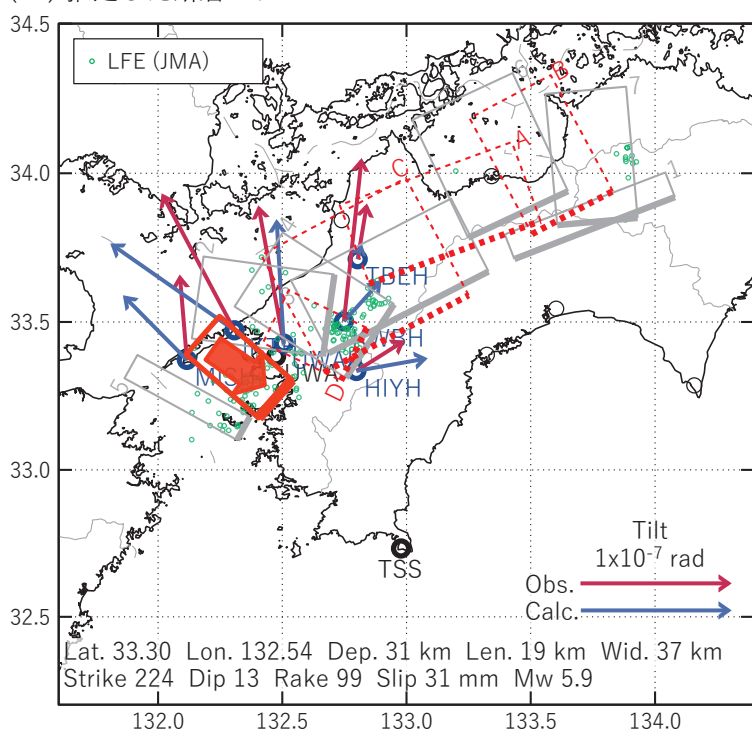
図8 2021/07/29-08/01AMの歪・傾斜変化 (図2,3[E]) を説明する断層モデル。
