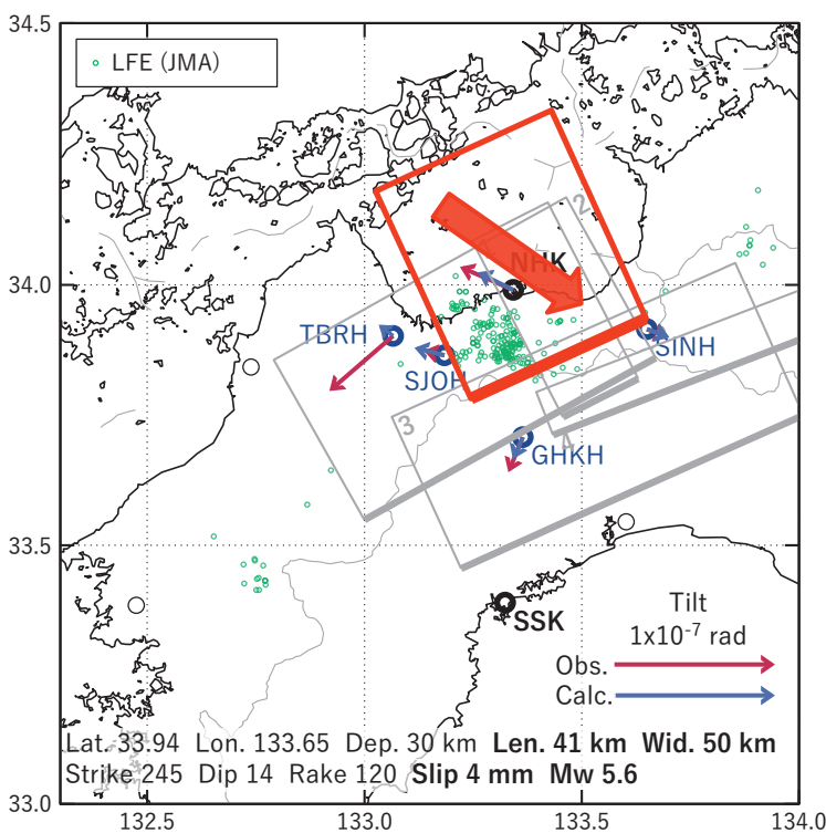
図3 2021/04/09 - 11AM の歪・傾斜変化 (図2[A]) を説明する断層モデル。
