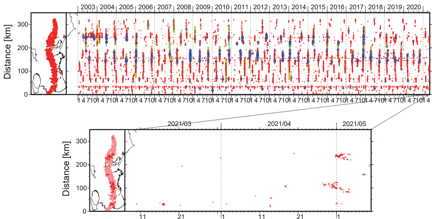
図1. 紀伊半島・東海地域における2003年1月～2021年5月9日までの深部低周波微動の時空間分布(上図). 赤丸はエンベロープ相関・振幅ハイブリッド法(Maeda and Obara, 2009)およびクラスタ処理(Obara et al., 2010)によって1時間毎に自動処理された微動分布の重心である. 青菱形は周期20秒に卓越する超低周波地震(Ito et al., 2007)である. 黄緑色の太線はこれまでに検出された短期的スロースリップイベント(SSE)を示す. 下図は2021年4月を中心とした期間の拡大図である. 4月27日～5月4日頃に三重・奈良県境付近から奈良県南部において活発な微動活動がみられた. この活動は三重・奈良県境付近で発生し, 南西方向への活動域の移動がみられた. 4月30日～5月4日頃には, 愛知県西部から中部においてやや活発な活動がみられた. この活動は愛知県西部で開始し, 東西両方向に活動域の拡大がややみられた. 4月13～14日頃には和歌山県中部から和歌山・奈良県境付近において, 4月17日頃には奈良・三重県境付近において, 4月30日～5月1日頃には和歌山県中部において, 5月7～8日頃には三重県北部において, それぞれごく小規模な活動がみられた.
