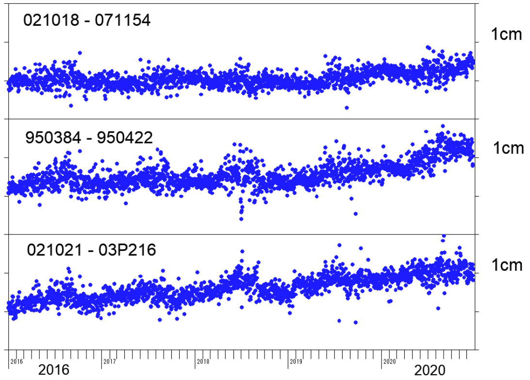
第3図 基線長変化 (2016年1月から2020年12月、直線トレンド・年周除去)
