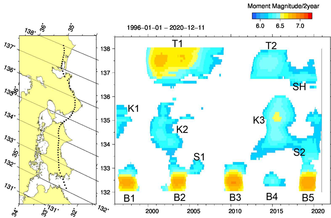
第2図 長期的スロースリップの規模分布（1996年から2020年12月） 2年間あたりの変化量から推定したモーメントマグニチュード。地域略号は第1図と同じ。
