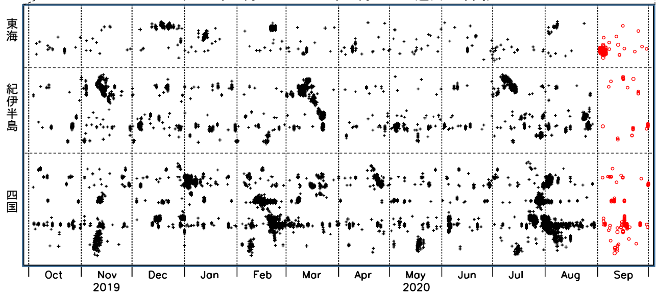
（2019年10月1日～2020年9月30日：過去1年間）
