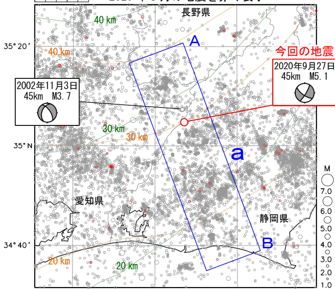
震央分布図 (1997年10月1日~2020年9月30日、 深さ0~60km、M≥1.0) 2020年9月の地震を赤く表示
