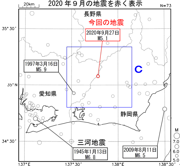
震央分布図 (1919年1月1日~2020年9月30日、 深さ0~100km、M≥5.0) 2020年9月の地震を赤く表示
