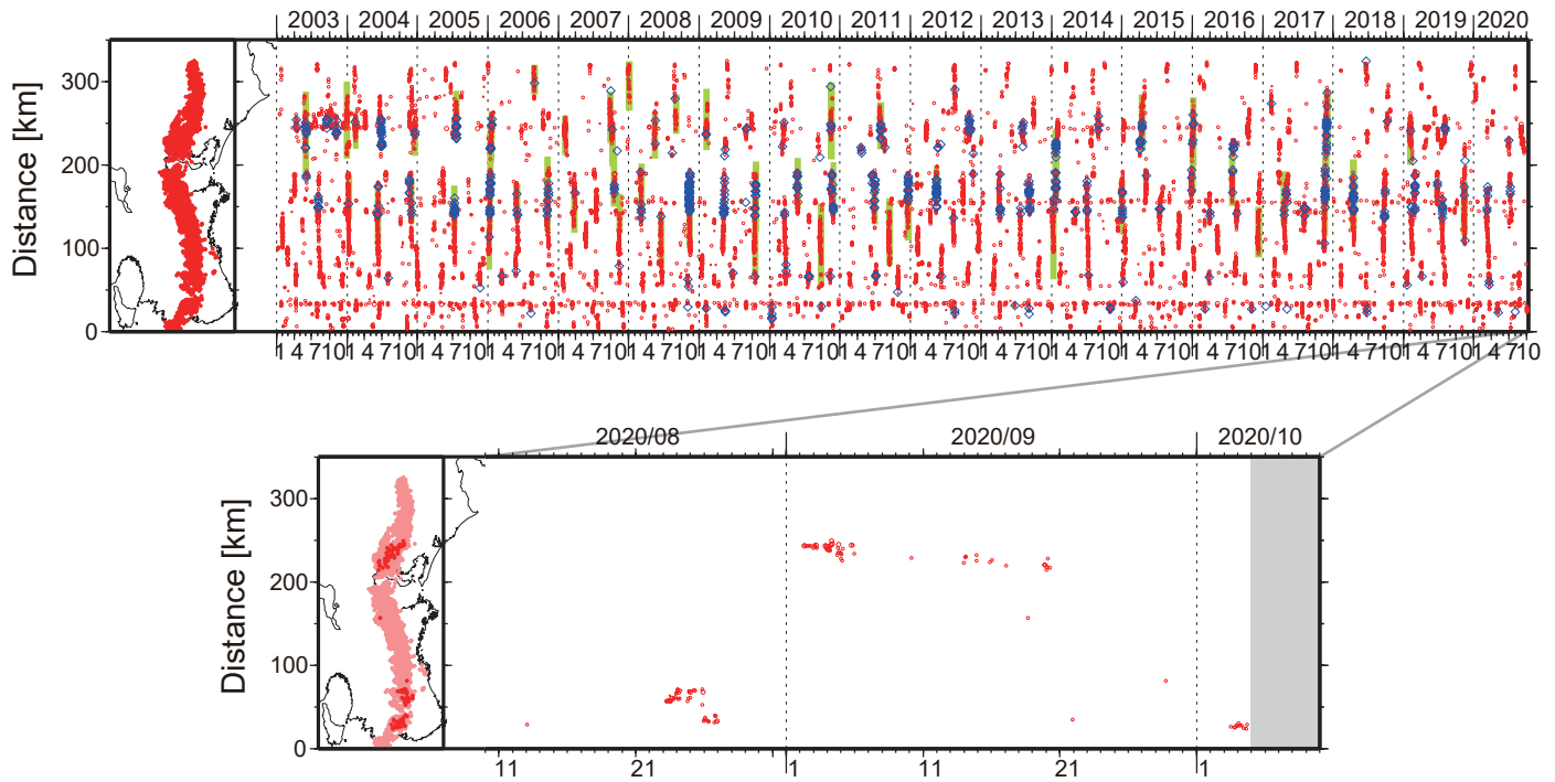
図1. 紀伊半島・東海地域における2003年1月～2020年10月4日までの深部低周波微動の時空間分布(上図). 赤丸はエンベロープ相関・振幅ハイブリッド法 (Maeda and Obara, 2009) およびクラスタ処理 (Obara et al., 2010) によって1時間毎に自動処理された微動分布の重心である. 青菱形は周期20秒に卓越する超低周波地震 (Ito et al., 2007) である. 黄緑色の太線はこれまでに検出された短期的スロースリップイベント (SSE) を示す. 下図は2020年9月を中心とした期間の拡大図である. 9月2～5日頃に愛知県中部から西部において、やや活発な微動活動がみられた. この活動は愛知県中部で開始し、西方向への活動域の拡大がみられた. この活動域の西側にあたる愛知県西部においては、9月13～17日頃に小規模な活動が、9月19～20日頃にはごく小規模な活動がみられた. 10月3日頃からは和歌山県中部において、微動活動が開始している.
