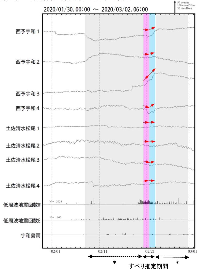
高知県から愛媛県で観測されたひずみ変化
