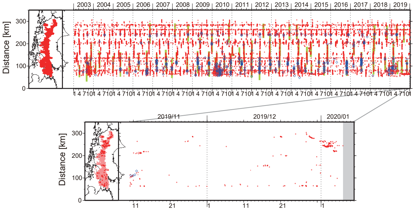
図1. 四国における2003年1月～2020年1月6日までの深部低周波微動の時空間分布(上図). 赤丸はエンベロープ相関・振幅ハイブリッド法 (Maeda and Obara, 2009) およびクラスタ処理 (Obara et al., 2010) によって1時間毎に自動処理された微動分布の重心である. 青菱形は周期20秒に卓越する超低周波地震 (Ito et al., 2007) である. 黄緑色太線は, これまでに検出された短期的スロースリップイベント (SSE) を示す. 下図は2019年12月を中心とした期間の拡大図である. 12月27日頃より徳島県東部において微動活動が開始したのち, 西方向への活動域の移動がみられた. その後, 1月1日頃からは徳島・香川・愛媛県境付近において活発化がみられ, さらに西方向への活動域の拡大がみられる. これ以外の活動として, 愛媛県中部において, 12月16～17日頃に小規模な活動がみられた. 香川県においては12月20～21日頃に, 愛媛県東部においては12月22日頃に, 愛媛県中部においては12月31日頃に, それぞれごく小規模な活動がみられた. 豊後水道においては, 12月21～22日頃にごく小規模な活動がみられ, 12月26～28日および12月29～31日頃にそれぞれ小規模な活動がみられた.
