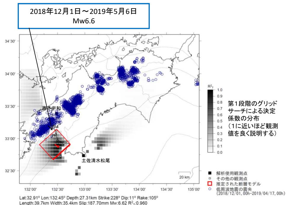
ひずみ変化から推定される断層モデル
