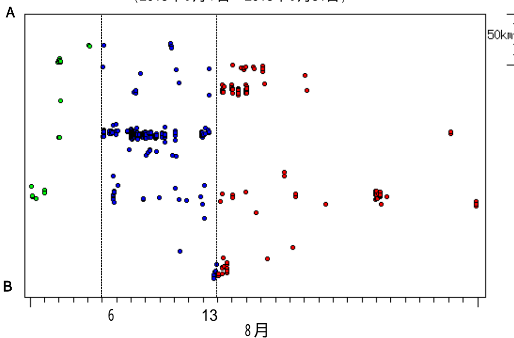
震央分布図の領域a内の時空間分布図(A - B投影) (2018年8月1日～2018年8月31日)
