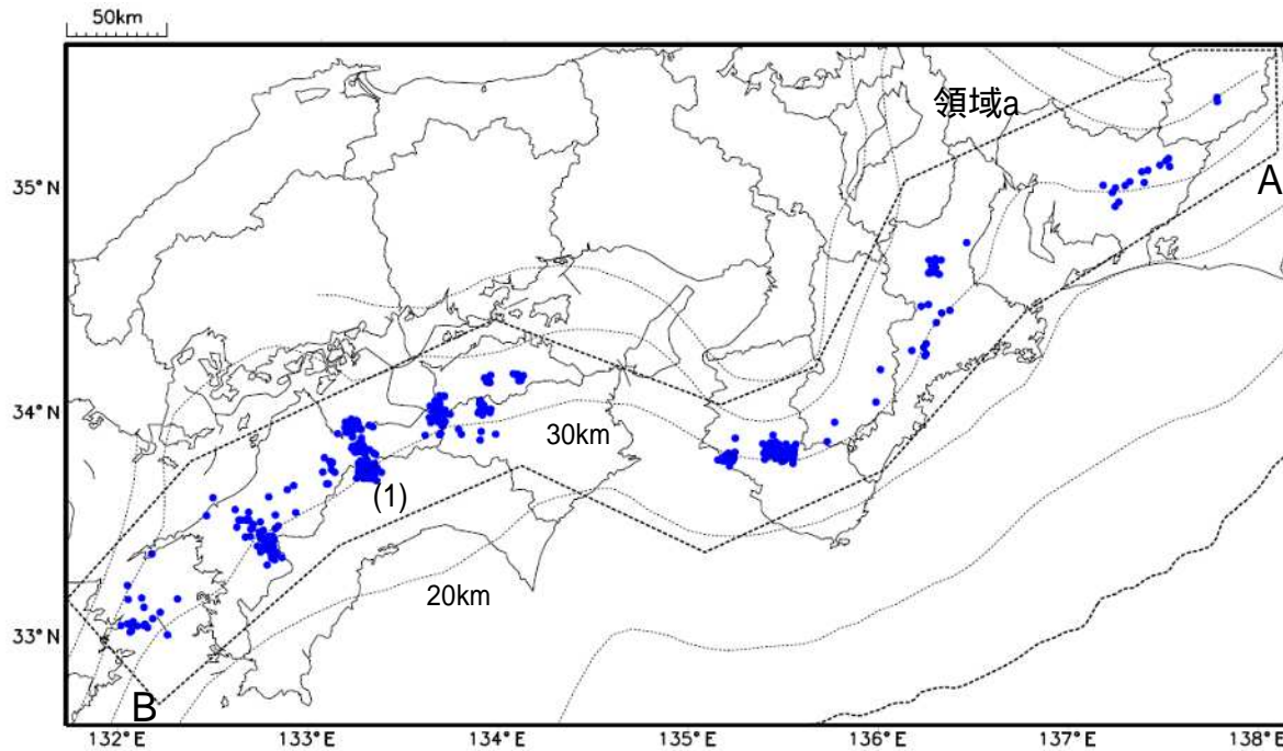
深部低周波地震(微動)の震央分布図(2018年8月1日～8月31日)
