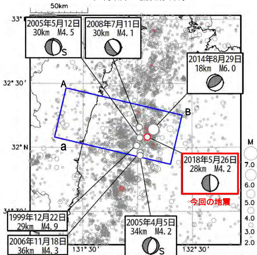
震央分布図 (1997年10月1日～2018年5月31日、M 2.0、深さ0～80km) 2018年5月以降の地震を赤く表示
