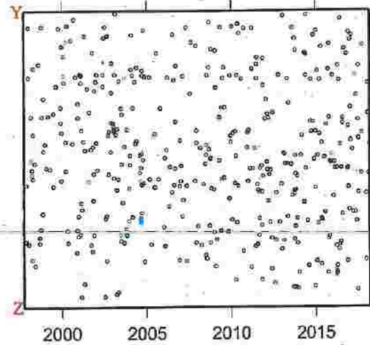
デクラスタ n=412
