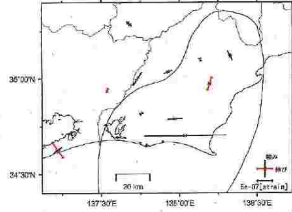
基準日：2017/12/14 比較日：2018/03/14
