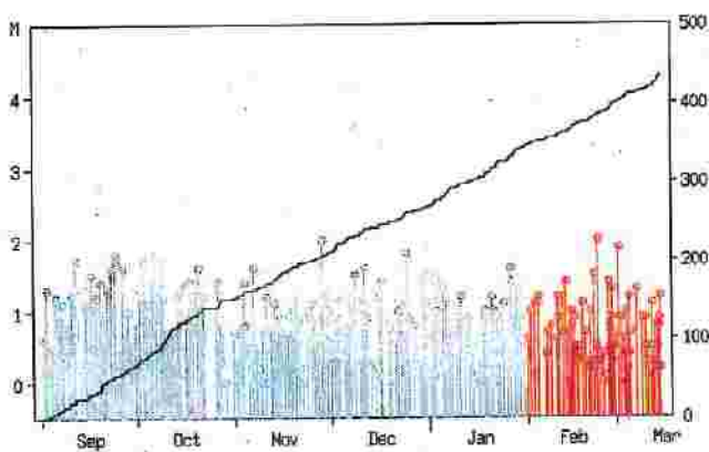
領域d内(四国)
