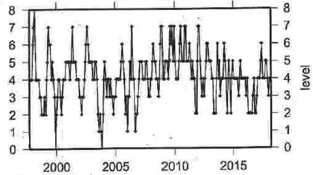
(5) 東海
