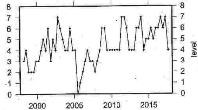
(6) 東南海
