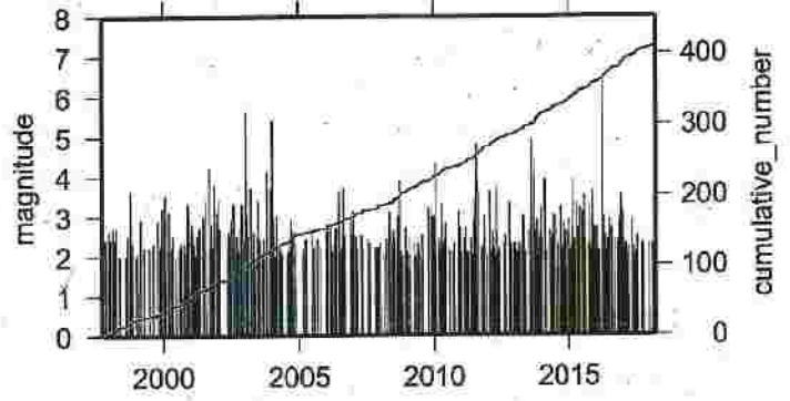
デクラスタ n=412
