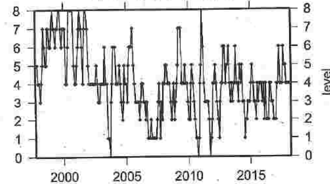
(14) 四国 (地殻内)
