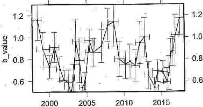
b 値 (地震数30個を15個ずつシフト)
