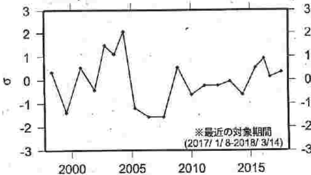
b 値 (地震数30個を15個ずつシフト)
