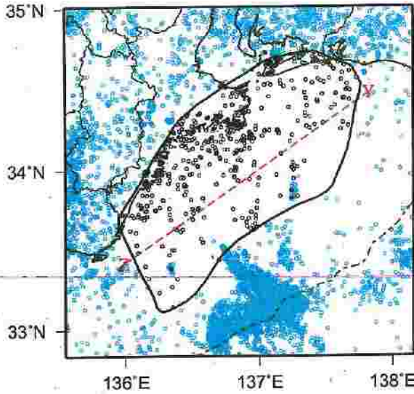
ノーマル n=525
