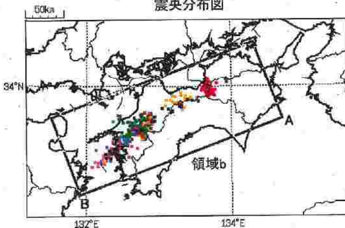
震央分布図
