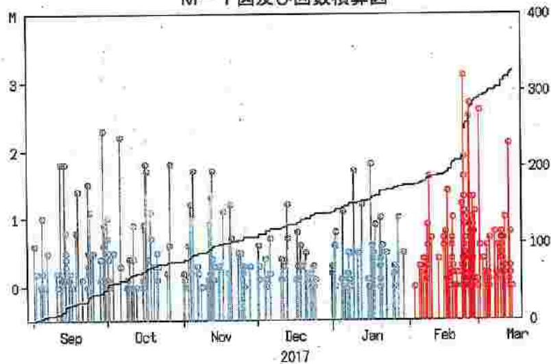
M-T図及び回数積算図
