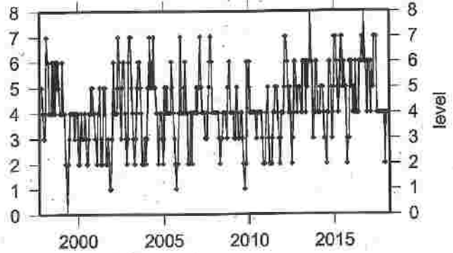
(11) 日向灘
