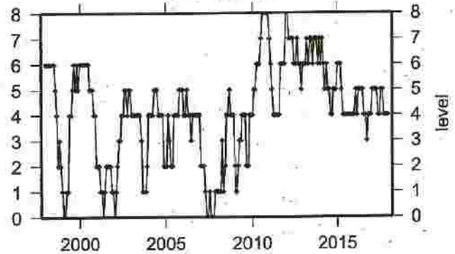
(4) 駿河湾
