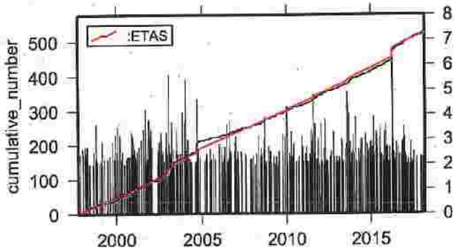
ノーマル n=525
