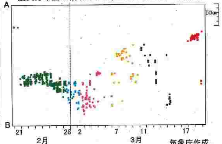
震央分布図の領域b内の時空間分布図(A-B投影)
