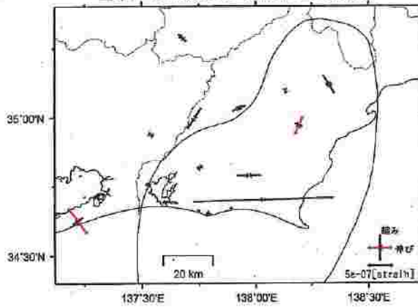
基準日：2017/12/01 比較日：2018/03/01
