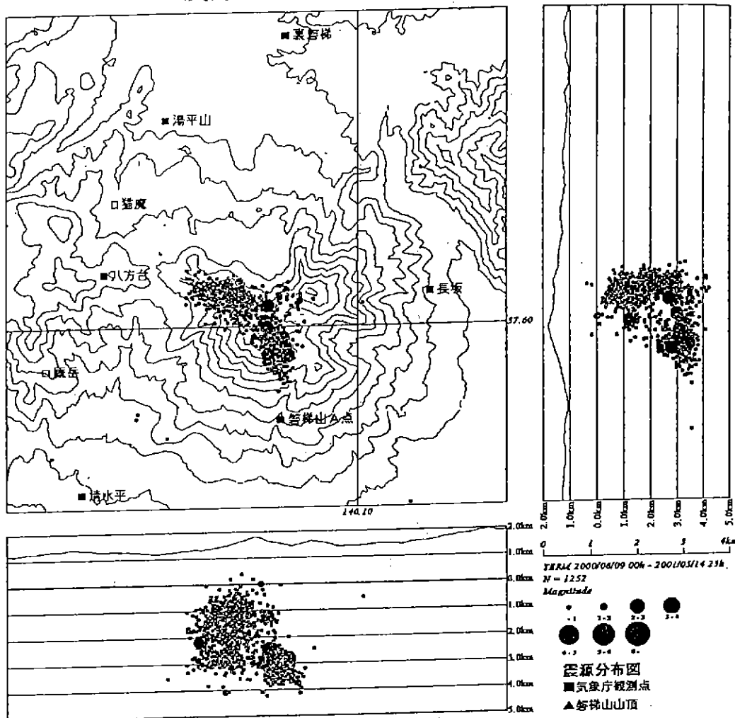
震源分布図 (2000.6.9-2001.5.14)
