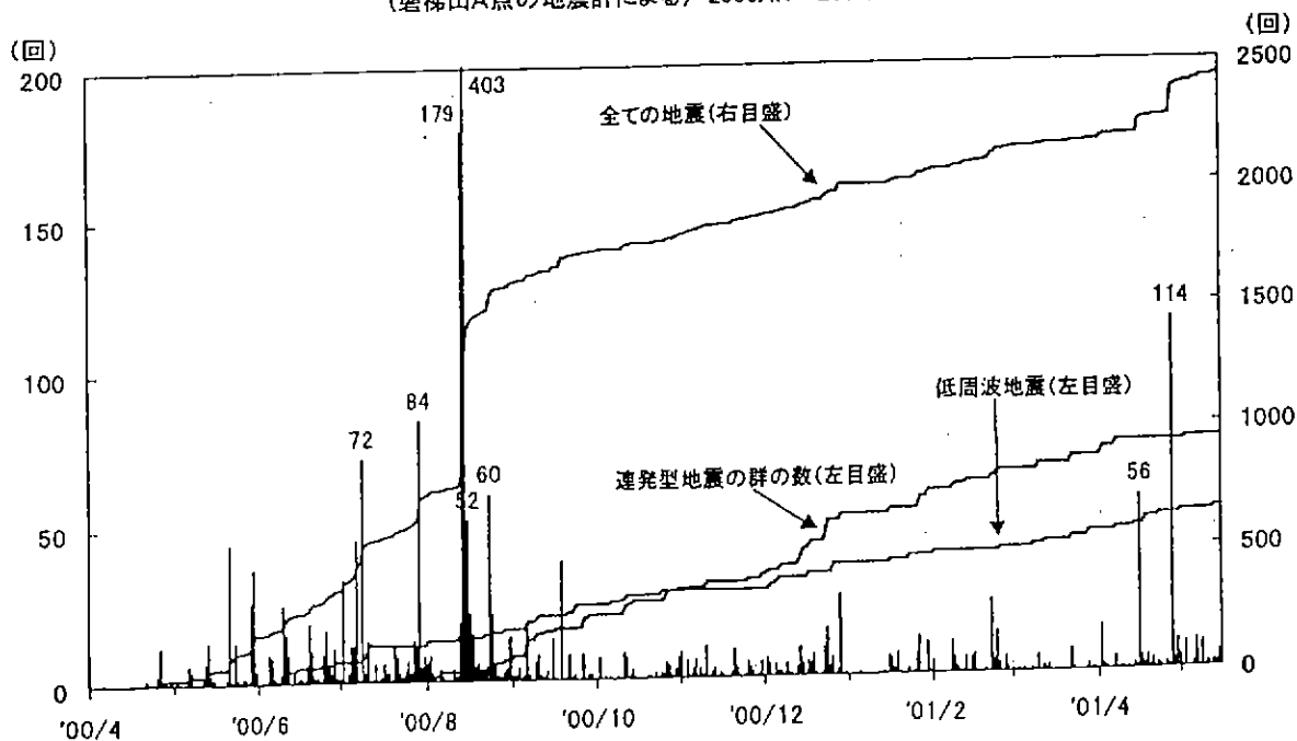
磐梯山の日別地震回数と積算回数グラフ (磐梯山A点の地震計による) 2000.4.1~2001.5.14
