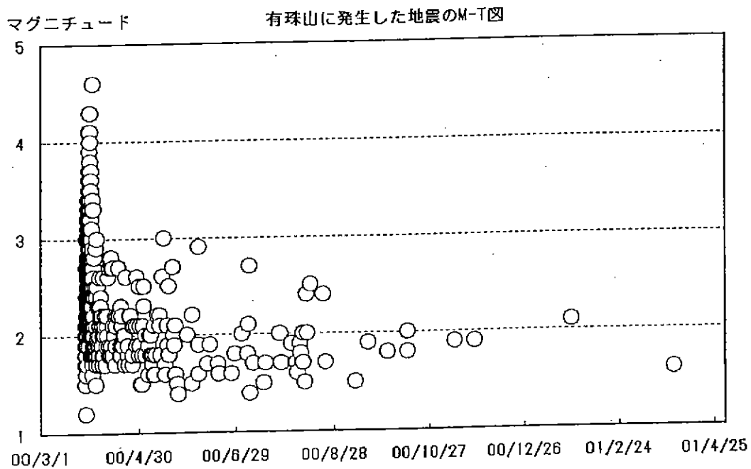
図5 気象庁A点で観測された火山性地震の発生状況 (2000年3月1日~2001年5月24日) 上段:日別地震回数の変化図 下段:M-T図
