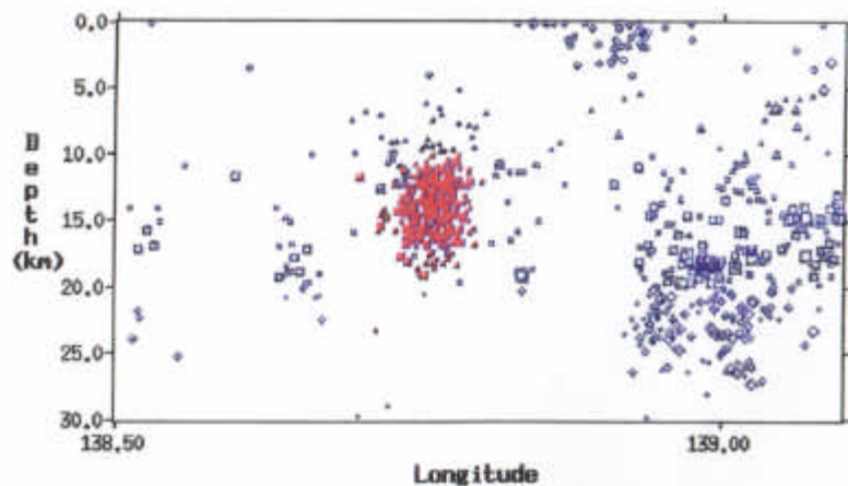
富士山周辺震源分布図 (2000/1/1~2001/2/1 05h:2000年7月未処理)
