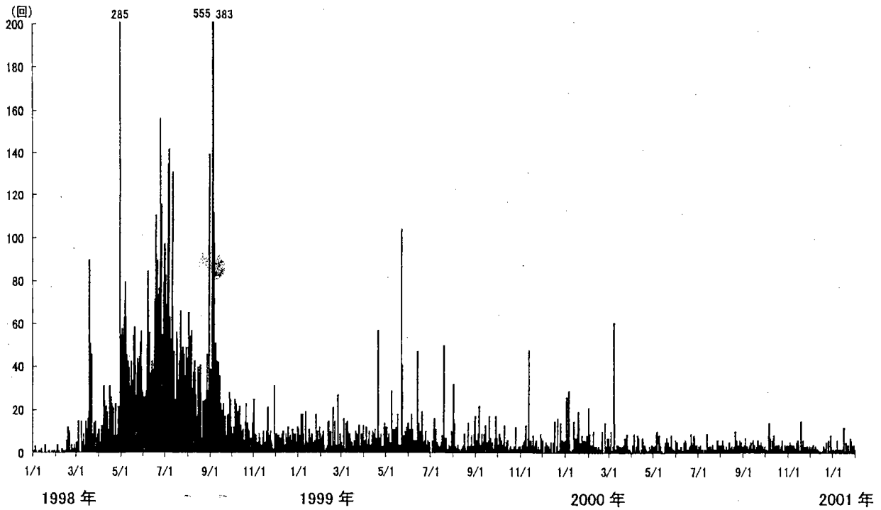
岩手山日別地震回数(東北大学松川観測点による)1998年1月1日～2001年1月31日
