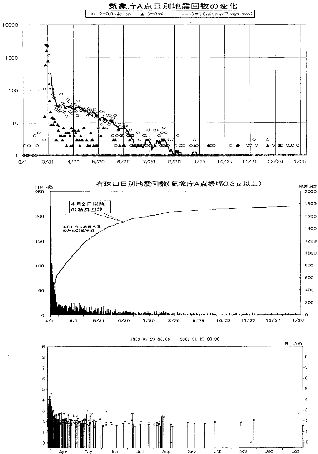
図6 気象庁A点で観測された火山性地震の発生状況(2000年3月~2001年1月) 上段:日回数変化図 中段:日別回数および積算曲線 下段:MT図
