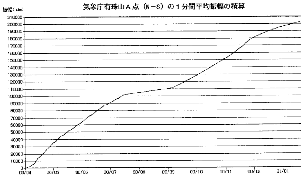
図4 気象庁A点NS成分で観測された噴火活動に伴う火山性微動の振幅レベルの推移 (2000年4月～2001年1月) 上段：特別最大振幅および周期の時間変化 下段：1分間平均振幅値の積算曲線
