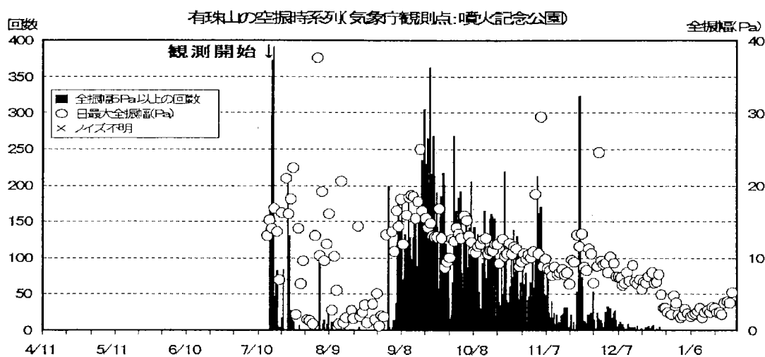
図2 空振パルスの特別回数および日別最大振幅の時系列図 (2000年4月～2001年1月, グラフ表示期間中に観測点変更を含む)
