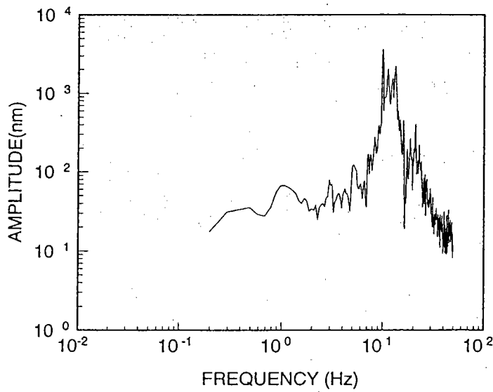
図 . 2000年8月1日に黒倉山から鬼ヶ城の直下で発生した単色地震(M0.2)の(a)波形例と(b)スペクトル. 卓越周波数は約10Hz
