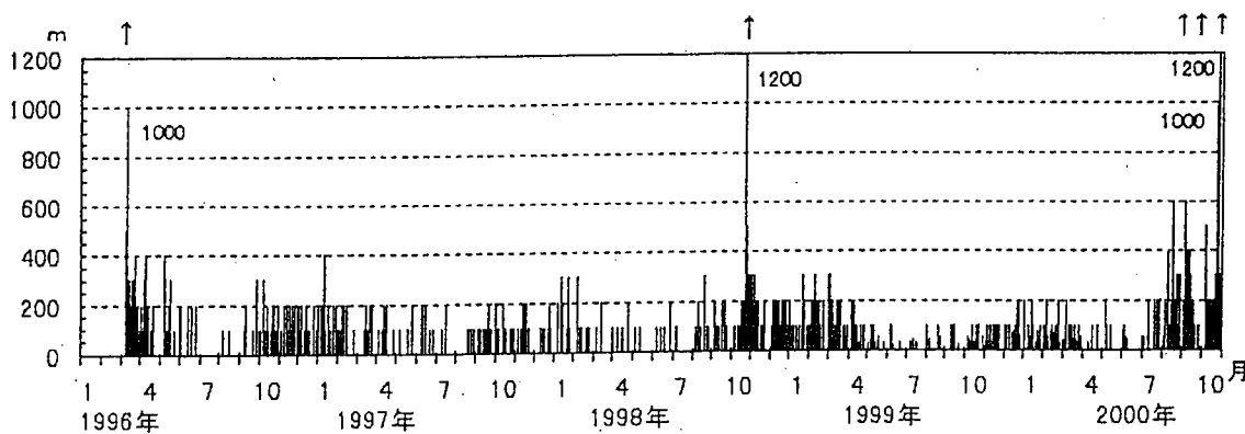
図5 北海道駒ヶ岳日別最高噴煙高度(1996.1.1-2000.10.30) ↑:噴火 本年7月以降、噴煙の多い状態が続いている
