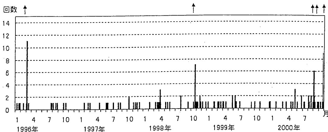
図4 北海道駒ヶ岳日別地震回数(1996.1.1-2000.10.30) ↑:噴火 火山性地震は9月4日の噴火直後から翌日にかけてやや増加したほかは、地震回数の少ない状態で推移した。
