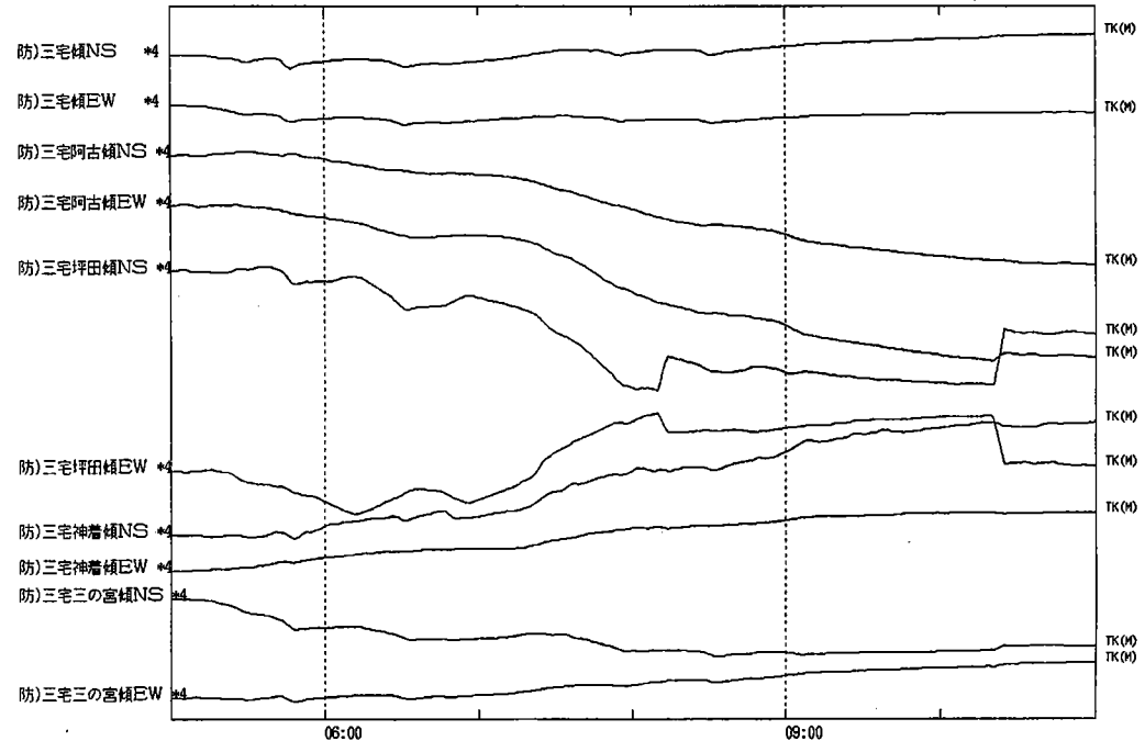
三宅島傾斜(防災科技研 補正分値) 2000/08/10 05:00 - 2000/08/10 11:00
